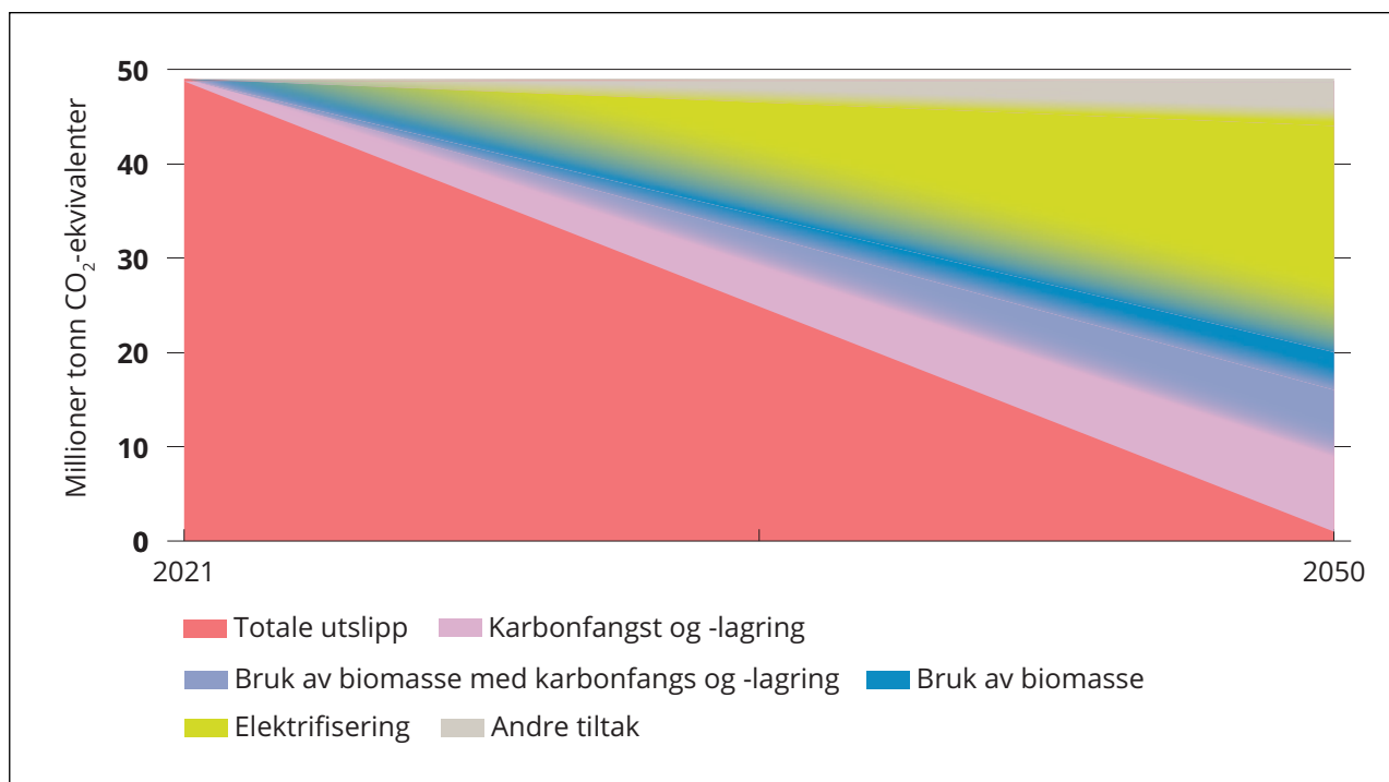
Figur 3.11 Fordeling av tiltak som elektrifisering, bruk av biomasse, karbonfangst og -lagring og andre tiltak for å redusere utslippene mot 2050.
