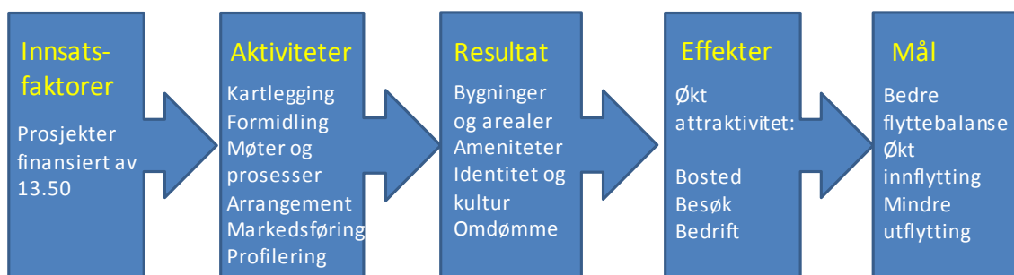
Figur 2: Programlogikk, enkel.
