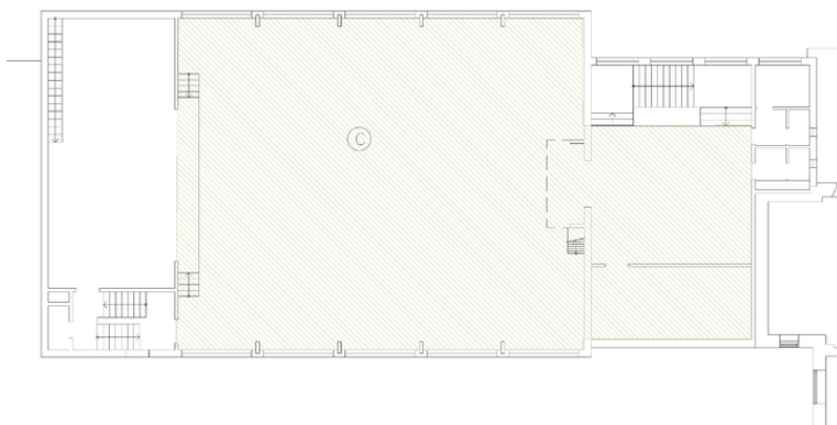
Plantegning 2. etasje med skravur for interiørvern. Opphavsrett: Statsbygg.
