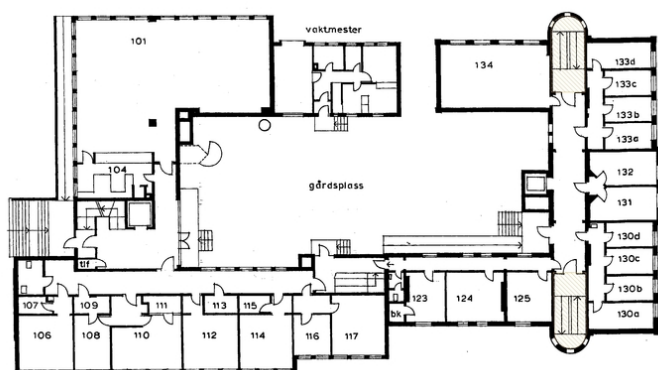
Plantegning 1. etg med skravur for vernet interiør. Opphavsrett: Statsbygg.
