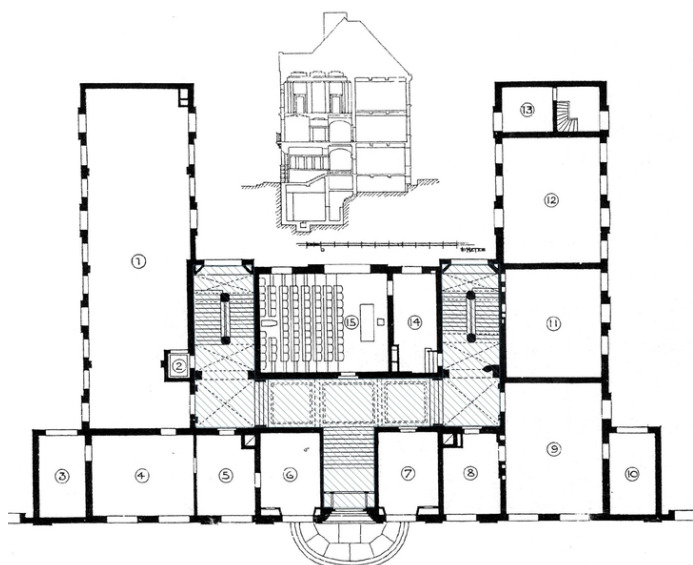
Plantegning 1. etg med skravur for fredet interiør. Opphavsrett: Statsbygg.
