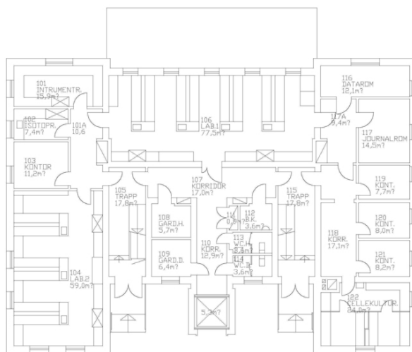
1. etg. Opphavsrett: NVH
