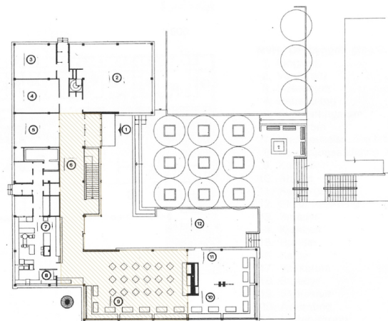
Plantegning 1. etg med skravur for vernet interiør. Opphavsrett: Statsbygg.
