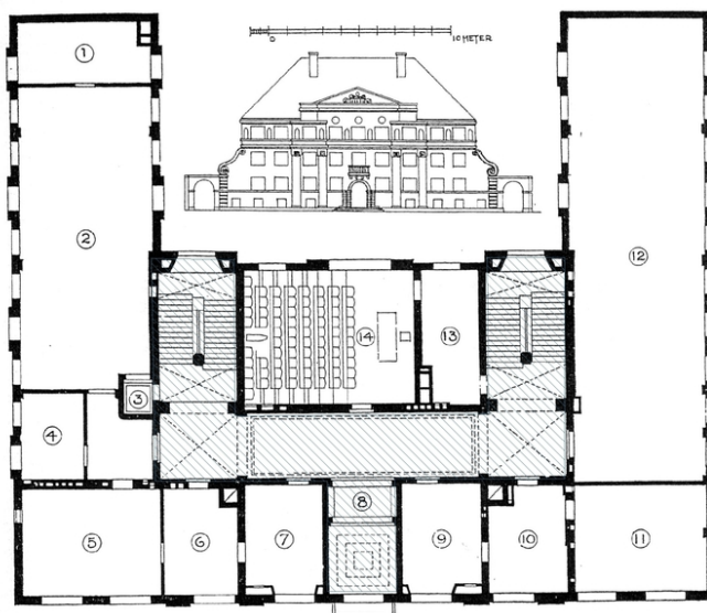
Plantegning 2. etg med skravur for fredet interiør. Opphavsrett: Statsbygg.
