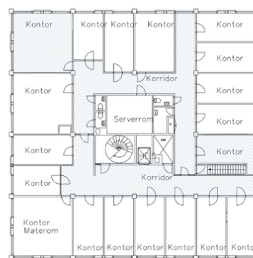
Plantegning 4. etg med skravur for vernet interiør. Opphavsrett: Statsbygg.
