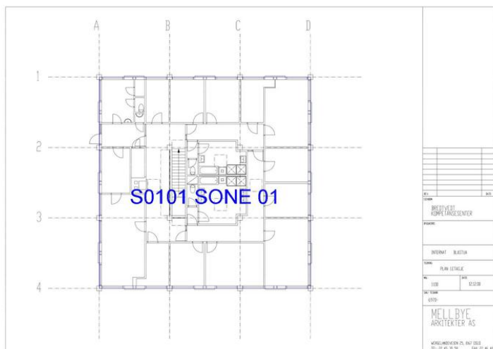
Plan 1. etajse. Opphavsrett: Statsbygg.
