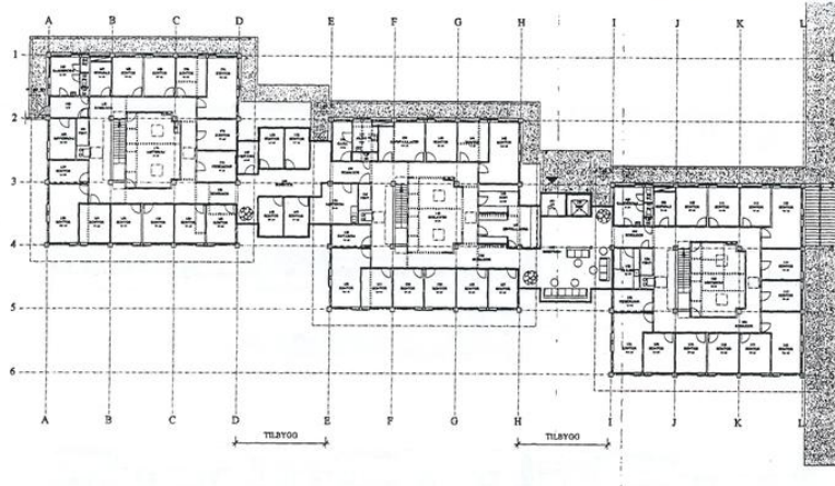
Plan 1. etasje Gul, grønn og rød med nye mellombygg Opphavsrett: Mellbye arkitekter as.
