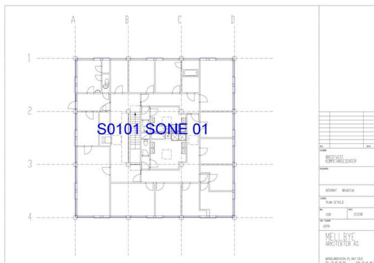
Plan først etasje. Opphavsrett: Statsbygg.
