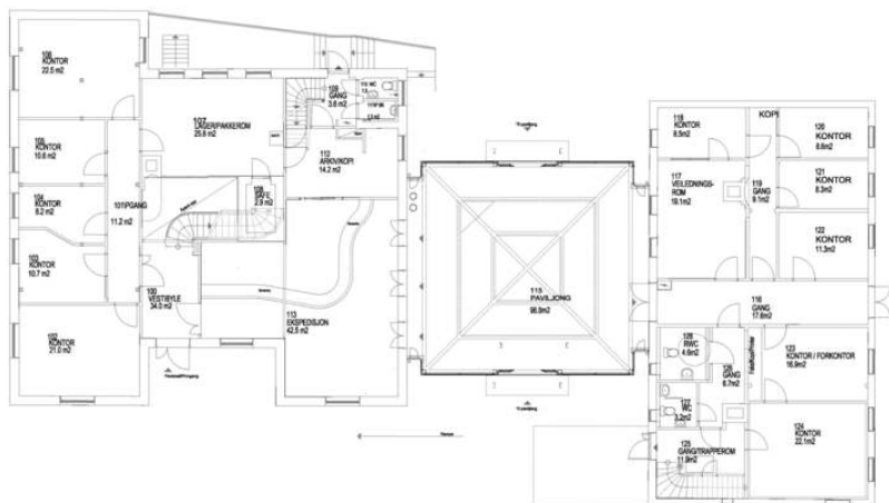
Plantegning 1. etasje Langesgt. 1 og 3. Opphavsrett: UiB.
