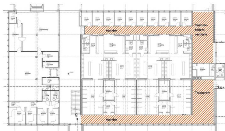
Plantegning 1. etasje. Vernesone interør: Inngangsparti med vindfang mot sørøst (nærmest svømmehallen) som er svømmehallens vestibyle, samt korridorer på begge sider av garderoberne. Opphavsrett: Statsbygg.
