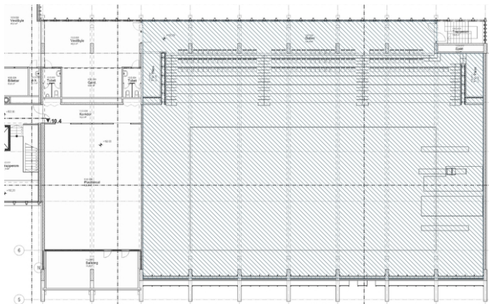
Plantegning 1. etasje med skravur for fredet interiør. Opphavsrett: Statsbygg.
