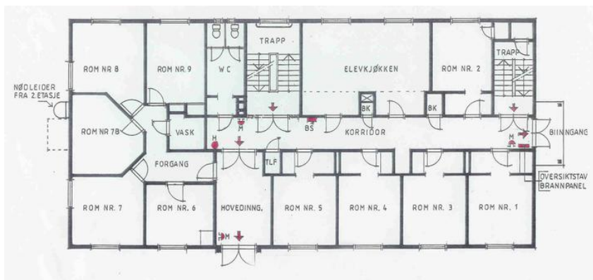
Plan 1.etg Opphavsrett: Vea
