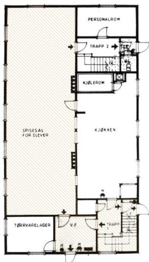
Plantegning 1.etg markert med skravur for vernet interiør. Opphavsrett: Statsbygg
