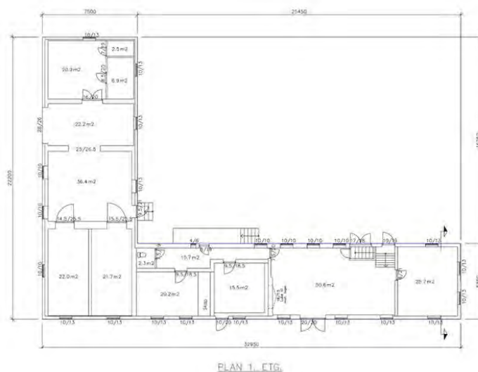
Plan første etasje. Opphavsrett: Statsbygg.
