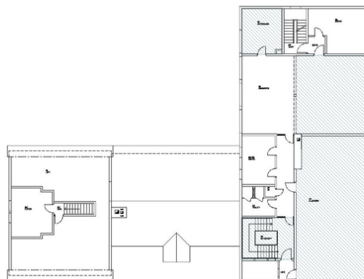
Plantegning 2. etasje med skravur for fredet interiør. Opphavsrett: Statsbygg.
