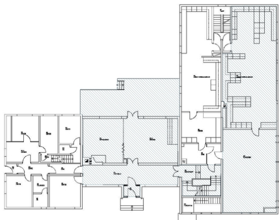
Plantegning 1. etasje med skravur for fredet interiør. Opphavsrett: Statsbygg.
