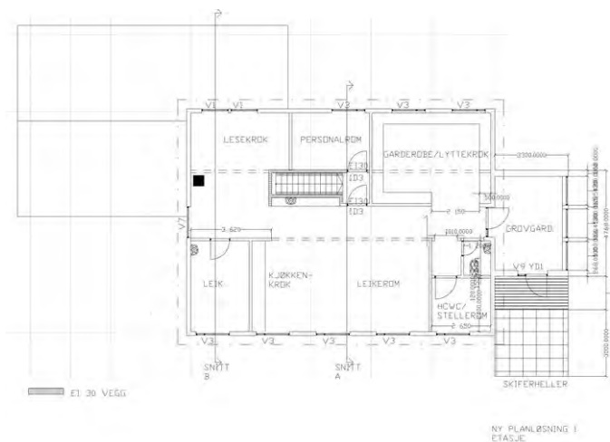
1. etasje, paviljong 6, barnehage. Opphavsrett: Statsbygg.
