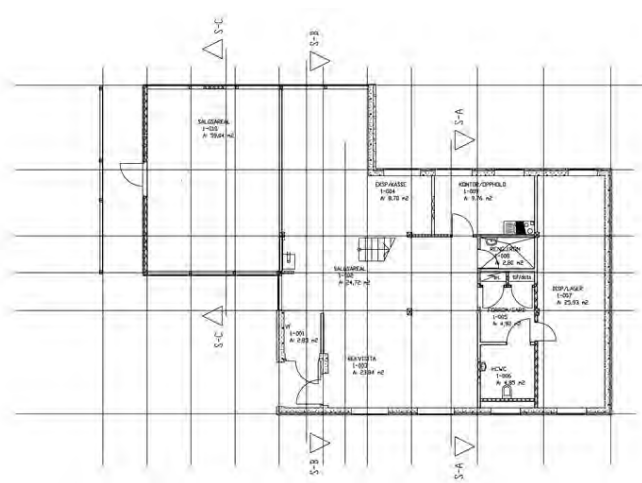
Plantegning sokkel, paviljong 1. Opphavsrett: Statsbygg.
