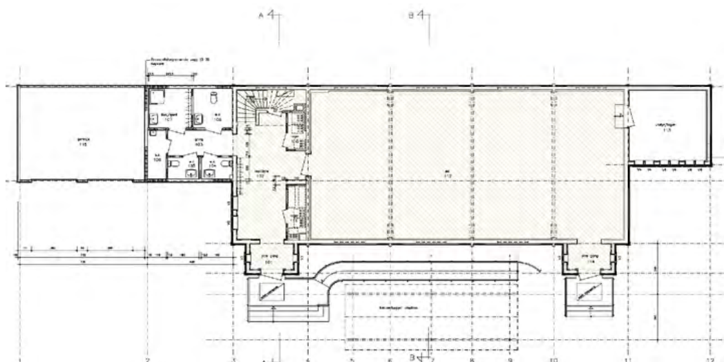
Plan 1. etasje med skravur for interiørværn. Opphavsrett: Statsbygg.
