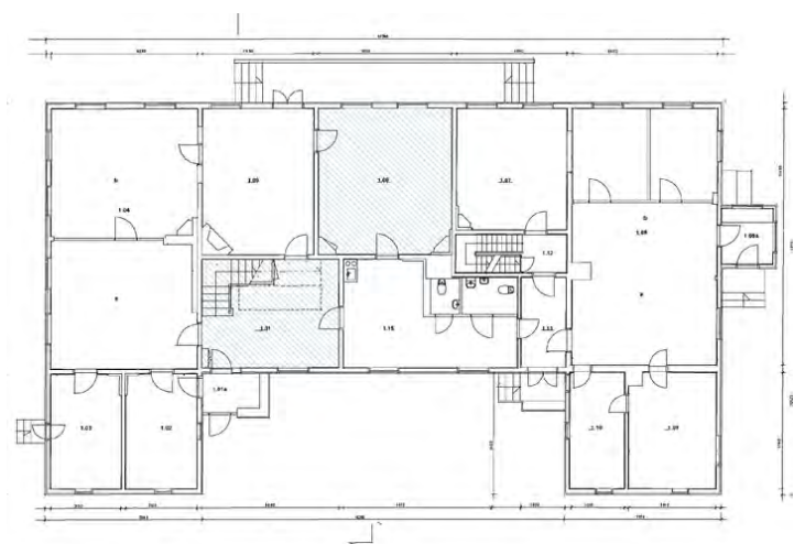
Plan 1. etg. med skravur for fredet interiør. Opphavsrett: Statsbygg.
