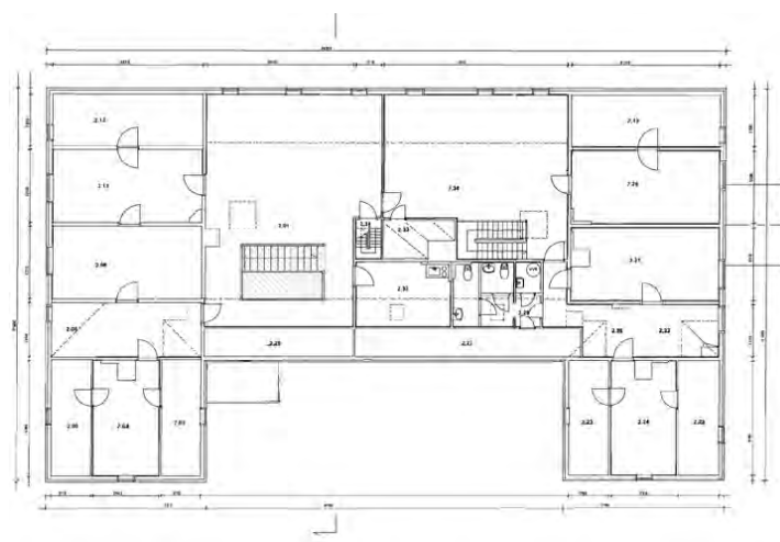
Plan 2. etg. med skravur for fredet interiør. Opphavsrett: Statsbygg.
