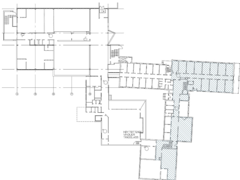
Plantegning 1. etasje med skravur for fredet interiør. Opphavsrett: Statsbygg.
