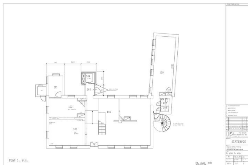
Plan 1. etasje. Opphavsrett: Statsbygg.
