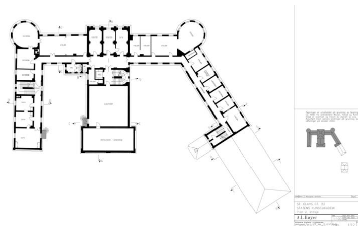
Plan 2. etasje. Opphavsrett: Statsbygg.
