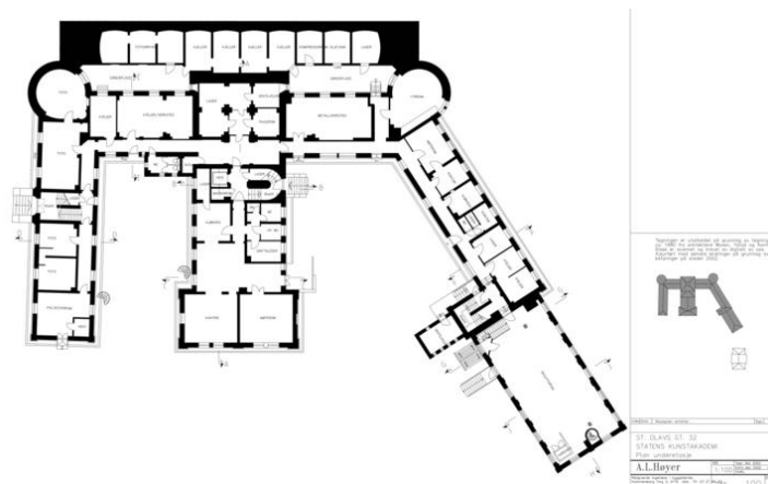
Plan Underetasje. Opphavsrett: Statsbygg.
