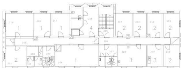
2. ETASJE BYGG A Mål 1:200
