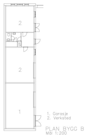
Plan 1. etasje. Opphavsrett: Statsbygg
