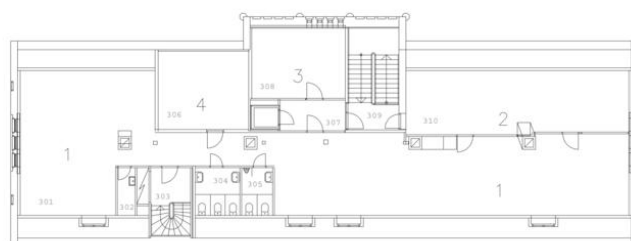
3. ETASJE BYGG A Mål 1:200
