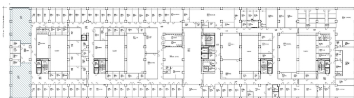
Plantegning 4. etasje med skravur for fredet interiør. Opphavsrett: Statsbygg.
