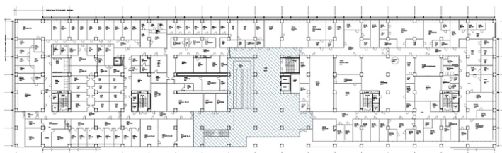
Plantegning 1. etasje med skravur for fredet interiør. Opphavsrett: Statsbygg.
