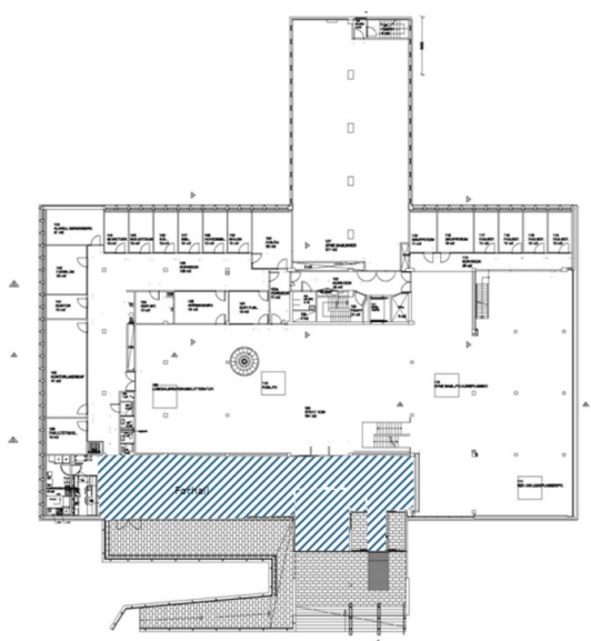
1.etg med interiørfredning markert med blå skravur. Opphavsrett: UiB.
