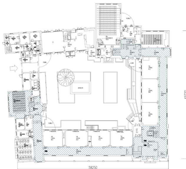
Plantegning 1. etasje med skravur for fredet interiør. Opphavsrett: Statsbygg.
