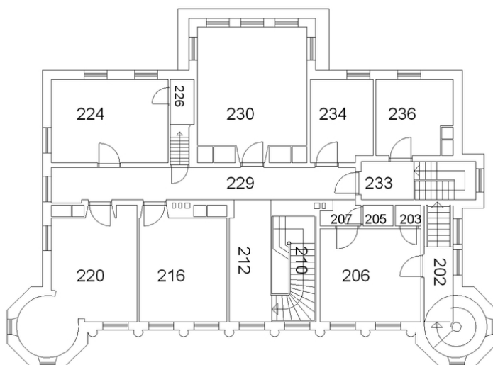
Plantegning 2. etg. Opphavsrett: Statsbygg.
