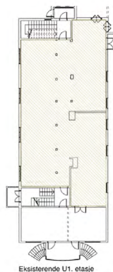
Plantegning U1. etasje Slottet med skravur for vernet interiør. Opphavsrett: Statsbygg.
