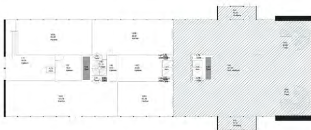
BL 10 Eilert Sunds Hus B 1 etg. med skravur for fredning. Opphavsrett: UiO.
