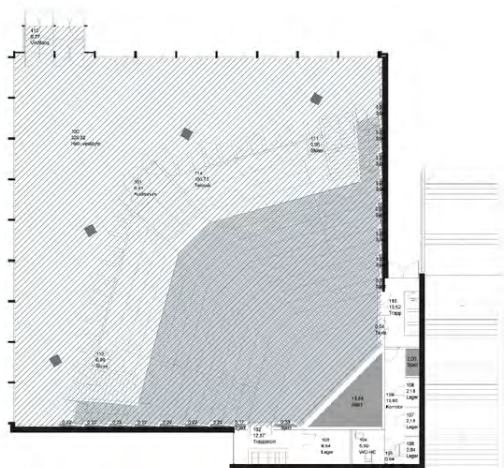
BL 15 Sophus Lies Aula 1 etg. med skravur for fredning. Opphavsrett: UiO.
