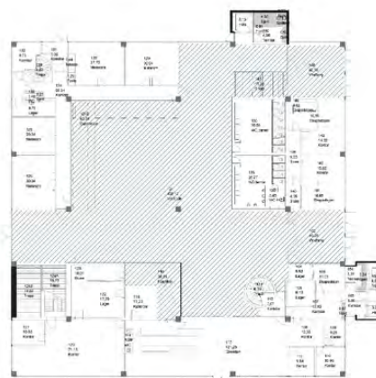
Chateau Neuf 1. etasje med skravur for interiørfredning. Opphavsrett: UiO.
