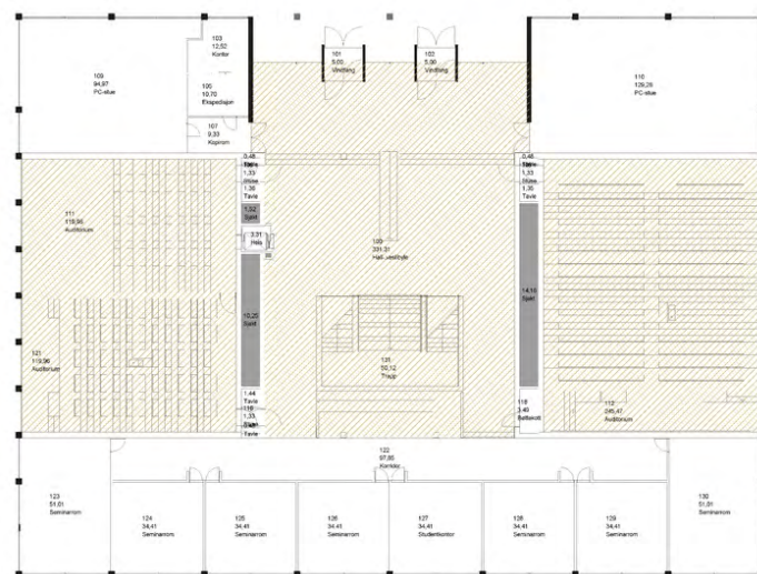
Plantegning 1. etasje Sophus Bugges Hus med skravur for vernet interior. Opphavsrett: Statsbygg.
