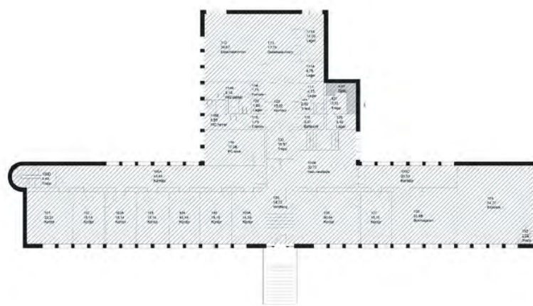
BL 26 Svein Rosselands hus 1. etasje med skravur for vern. Opphavsrett: UiO.
