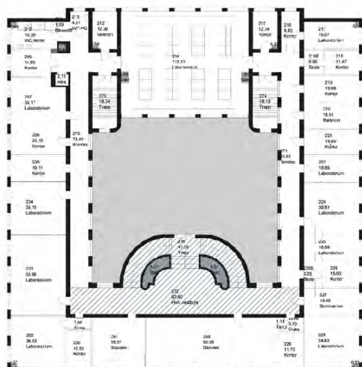
BL 25 Farmasøytisk 2 etg. med skravur for fredning. Opphavsrett: UiO.
