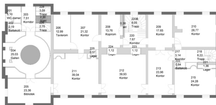
Plantegning 2. etasje. Opphavsrett: Statsbygg.
