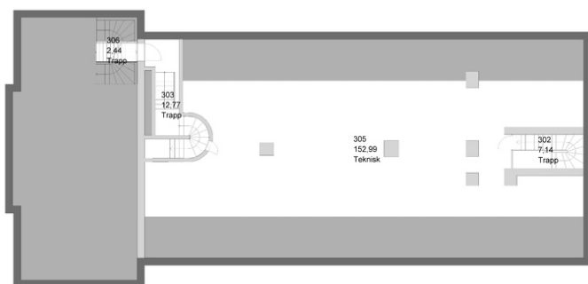
Plantegning 3. etasje. Opphavsrett: Statsbygg.
