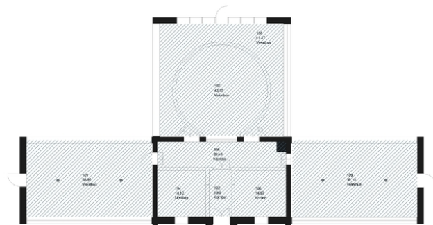
TØ 07 Victoria-Regia 1. etasje med skravur som vist på plantegning. Opphavsrett: UiO.
