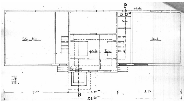
Låvens (østfløyens) opprinnelige planløsning og bruk, 1. etg. Fra v: vognskjul, stall, fjøs, bod. Opphavsrett: UiO.
