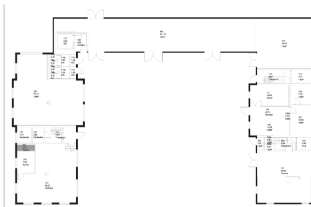
Plantegning 1. etg, alle fløyer. Opphavsrett: UiO.
