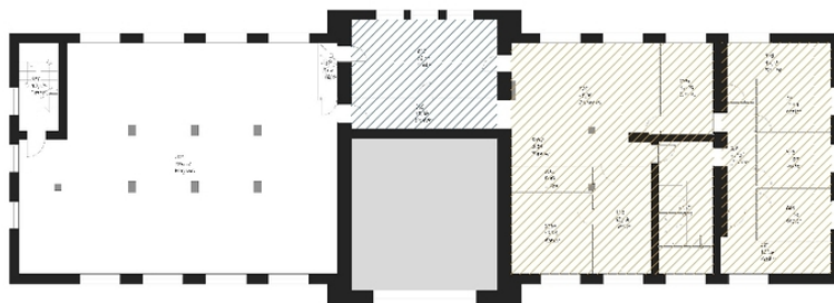
TØ03 Botanisk Museum 2. etasje med skravur for Vk1 og Vk2 på interiør. Opphavsrett: UiO.
