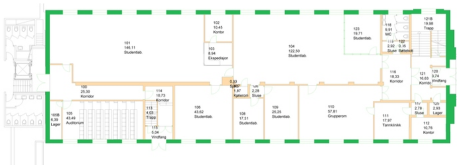
Plantegning 1. etg. Opphavsrett: UiO.
