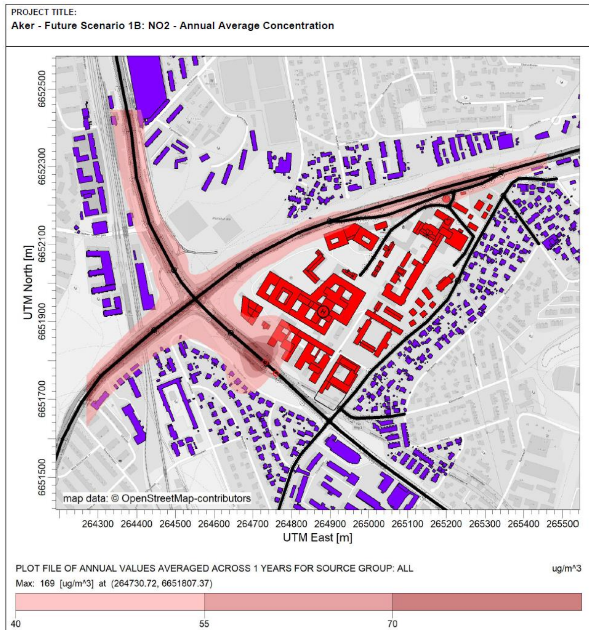
Figur 31. Luftsonerkart som viser modellerte konsentrasjoner av nitrogendioksid (NO 2 ) for området ved Aker sykehus ved 2-3 meters høyde for planalternativ 1B. Rød sone tilsvarer overskridelse av grensen på 40 µg/m 3 årsmiddel, i henhold til Retningslinje for behandling av luftkvalitet i arealplanlegging (T-1520) (Miljøverndepartementet, 2012).
