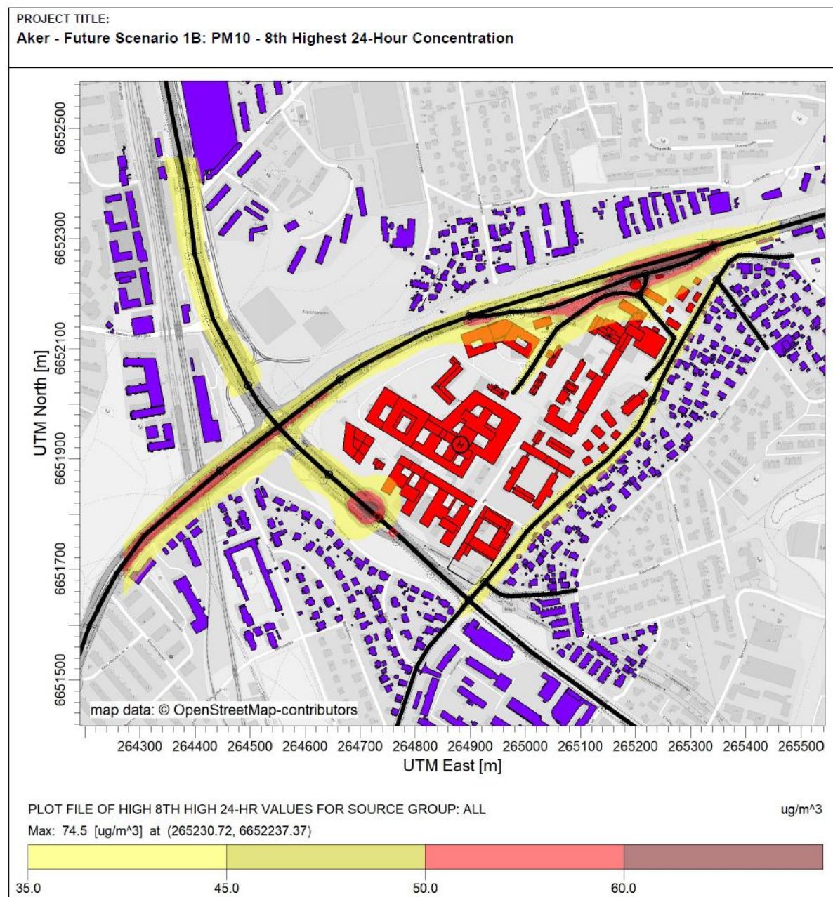
Figur 30. Luftsonekart som viser modellerte konsentrasjoner av svevestøv (PM 10 ) for området ved Aker sykehus ved 2-3 meters høyde for planalternativ 1B. Gul og rød sone for PM 10 tilsvarer maksimum 7 overskridelser av grensene på henholdsvis 35 og 50 µg/m 3 , i henhold til Retningslinje for behandling av luftkvalitet i arealplanlegging (T-1520) (Miljøverndepartementet, 2012).
