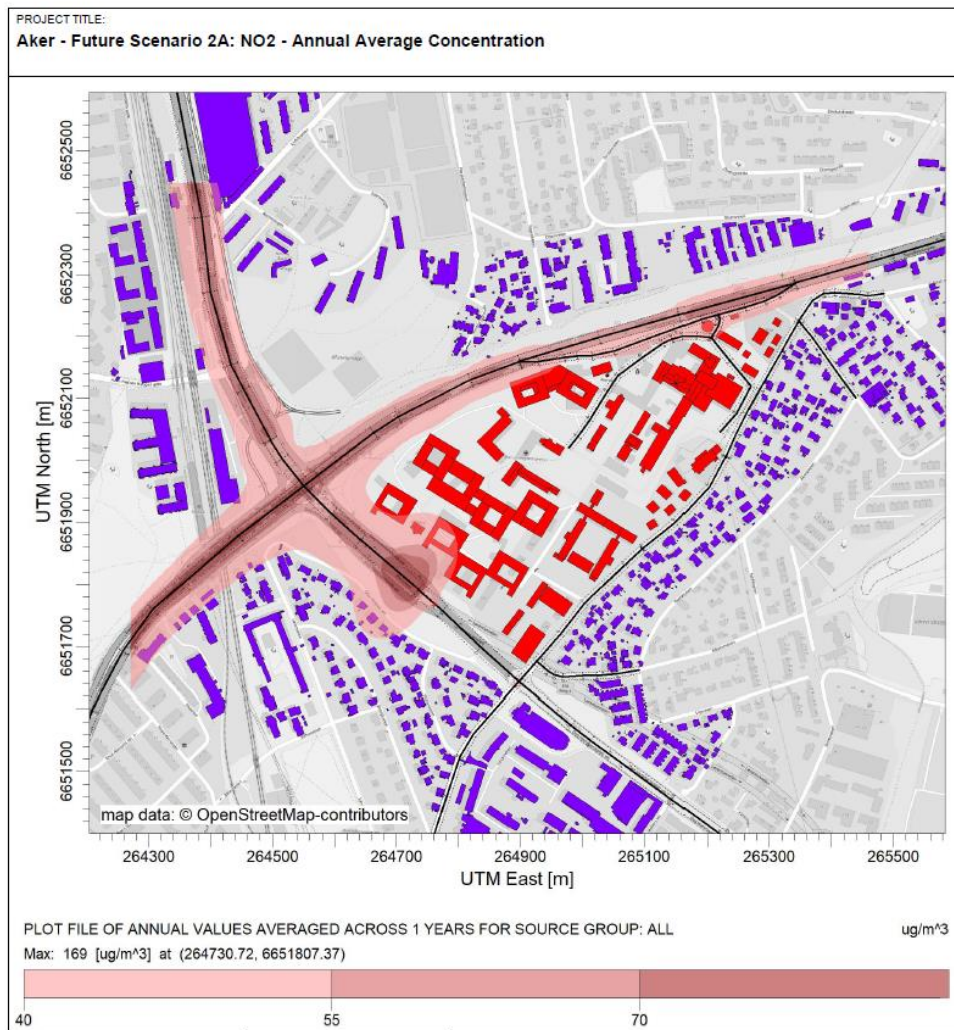
Figur V1- 8. Luftsonekart som viser modellerte konsentrasjoner av nitrogendioksid (NO 2 ) for området ved Aker sykehus ved 2-3 meters høyde for planalternativ 2A med støyskjerm mot Ring 3. Rød sone tilsvarer overskridelse av grensen på 40 µg/m 3 årsmiddel, i henhold til Retningslinje for behandling av luftkvalitet i arealplanlegging (T-1520) (Miljøverndepartementet, 2012).
