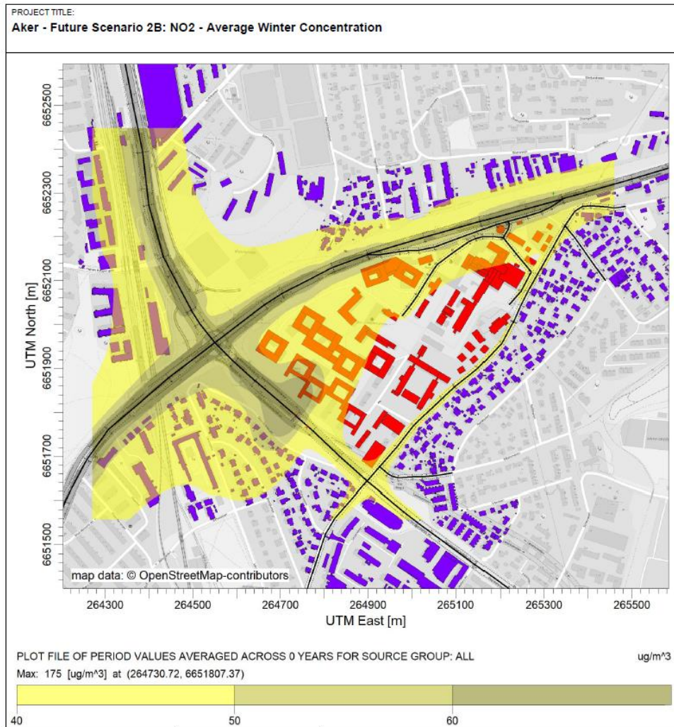
Figur V1- 12. Luftsonekart som viser modellerte konsentrasjoner av nitrogendioksid (NO 2 ) for området ved Aker sykehus ved 2-3 meters høyde for planalternativ 2B med støyskjerm mot Ring 3. Gul sone tilsvarer overskridelse av grensen på 40 µg/m 3 vintermiddel, i henhold til Retningslinje for behandling av luftkvalitet i arealplanlegging (T-1520) (Miljøverndepartementet, 2012).
