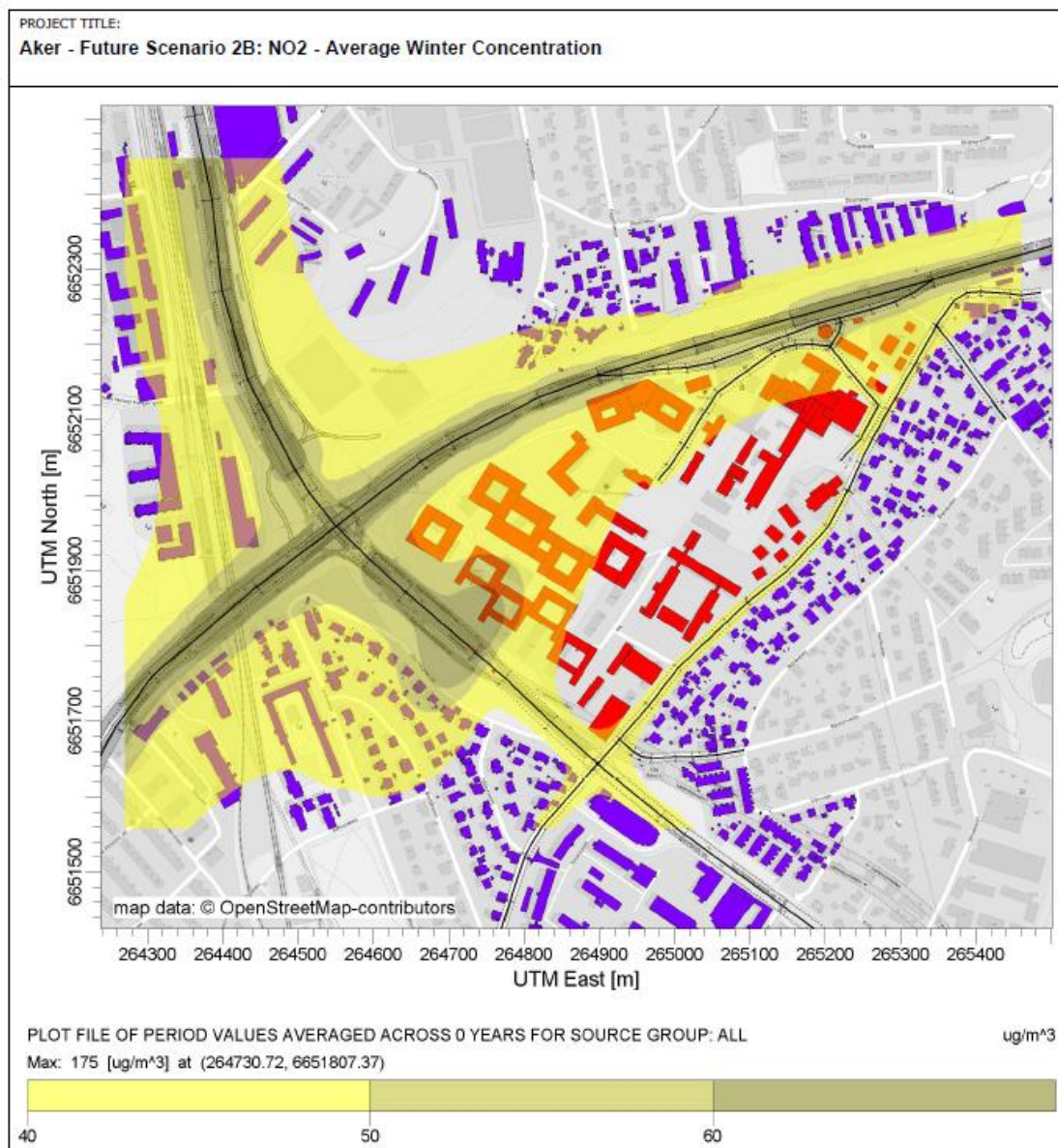
Figur 38. Luftsonerkart som viser modellerte konsentrasjoner av nitrogendioksid (NO 2 ) for området ved Aker sykehus ved 2-3 meters høyde for planalternativ 2B. Gul sone tilsvarer overskridelse av grensen på 40 µg/m 3 vintermiddel, i henhold til Retningslinje for behandling av luftkvalitet i arealplanlegging (T-1520) (Miljøverndepartementet, 2012).
