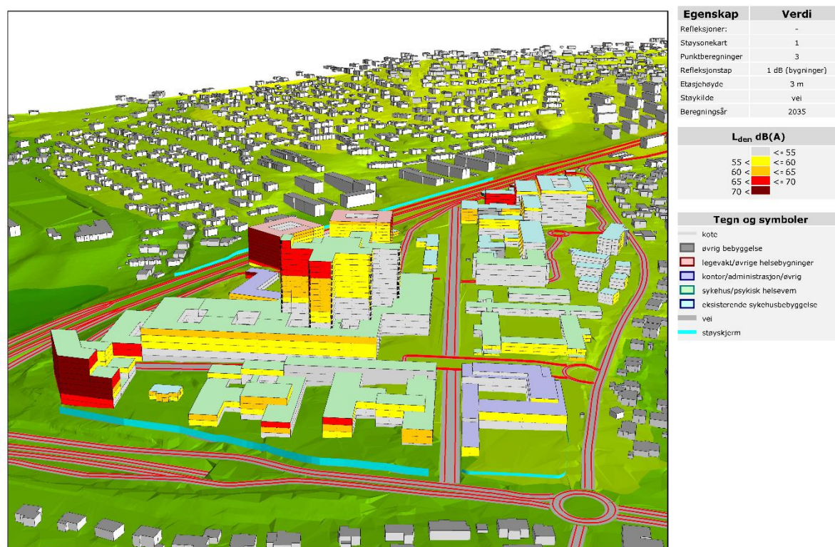
Figur 43. Støysonekart L den planalternativ 1A. Beregningshøyde 1,5 meter. (Rambøll Norge AS, 2019)
