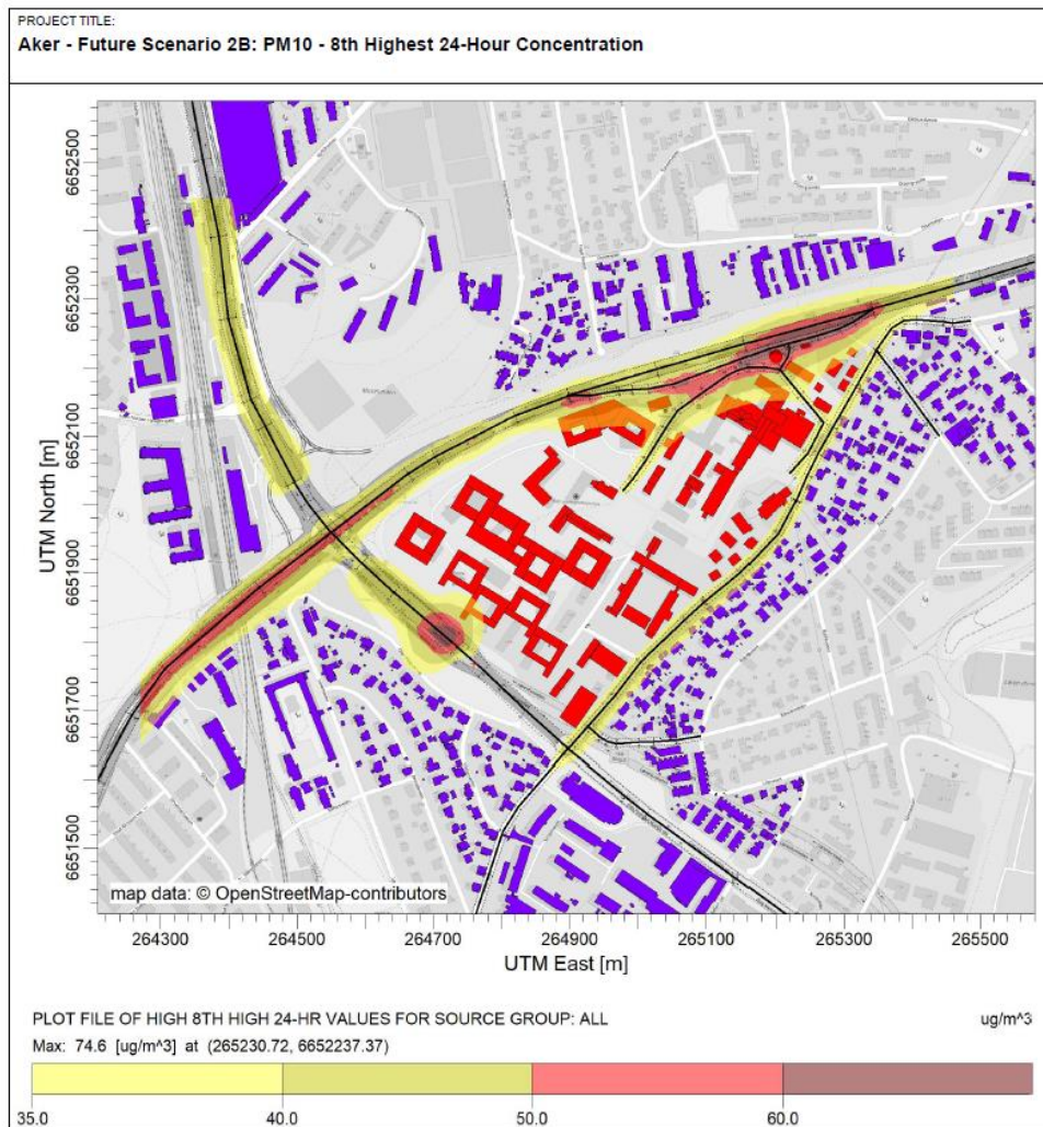
Figur V1- 10. Luftsonekart som viser modellerte konsentrasjoner av svevestøv ( \text{PM}_{10} ) for området ved Aker sykehus ved 2-3 meters høyde for planalternativ 2B med støyskjerm mot Ring 3. Gul og rød sone for \text{PM}_{10} tilsvarer maksimum 7 overskridelser av grensene på henholdsvis 35 og 50 \mu\text{g}/\text{m}^3 , i henhold til Retningslinje for behandling av luftkvalitet i arealplanlegging (T-1520) (Miljøverndepartementet, 2012)
