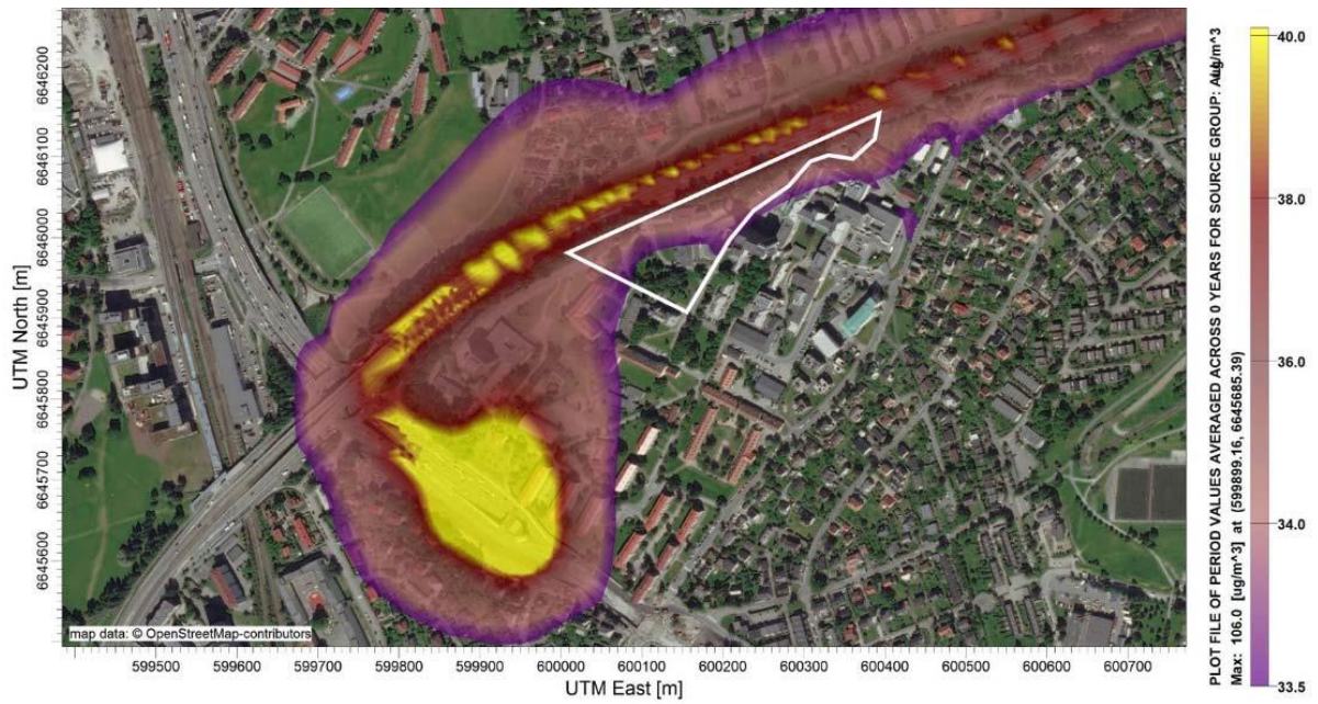
Figur 23. NO 2 vintermiddelkonsentrasjoner (µg/m 3 ) for 0-alternativet. Gul sone inntreffer når vintermiddelet overskrider 40 µg/m 3 . Merk at laveste verdi på skalaen er ulik laveste verdi for NO 2 årsmiddel (Figur 22). Planområdet for Oslo storbylegevakt er markert med hvitt omriss. (COWI AS, 2018)
