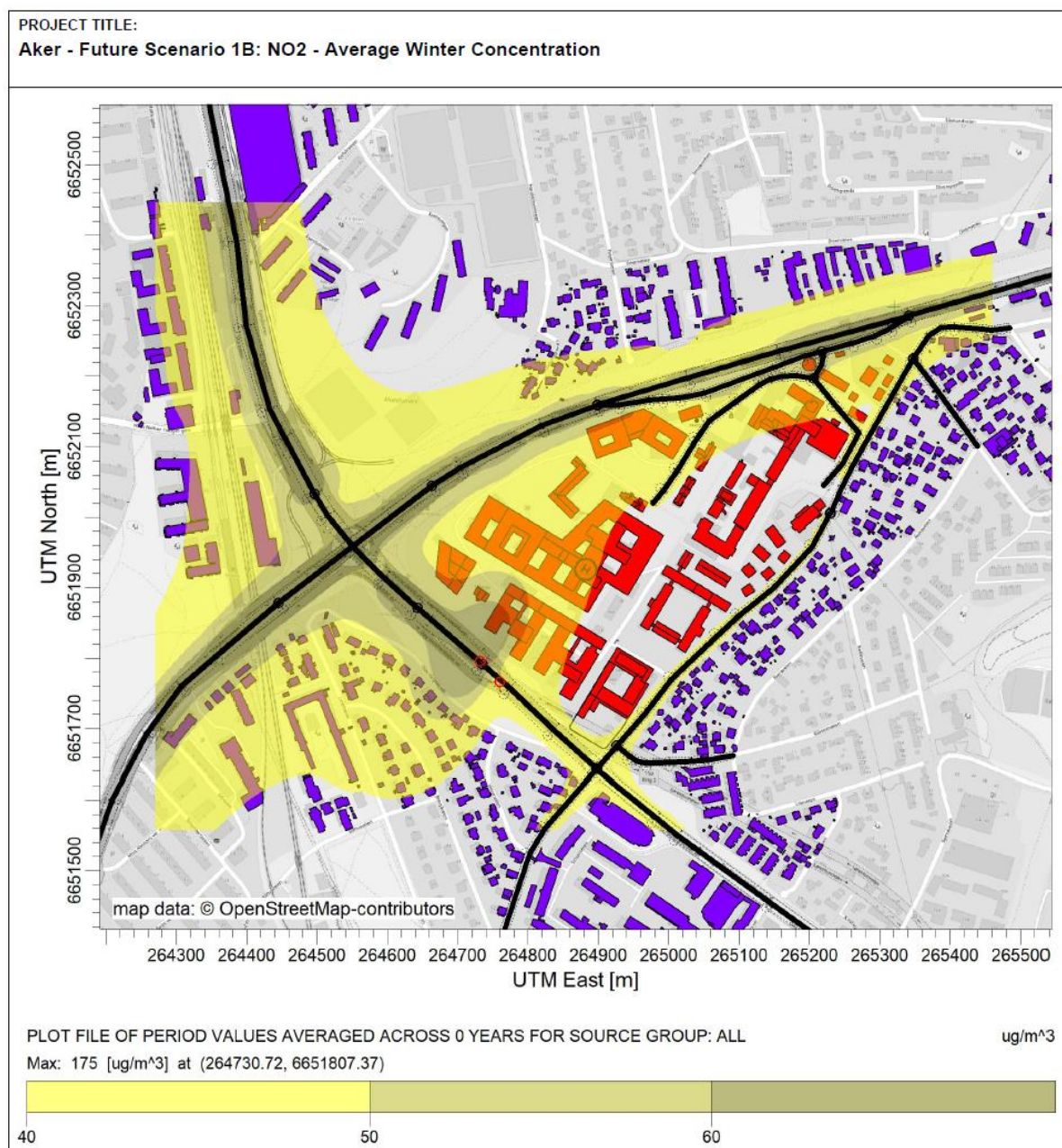
Figur 32. Luftsonekart som viser modellerte konsentrasjoner av nitrogendioksid (NO 2 ) for området ved Aker sykehus ved 2-3 meters høyde for planalternativ 1B. Gul sone tilsvarer overskridelse av grensen på 40 µg/m 3 vintermiddel, i henhold til Retningslinje for behandling av luftkvalitet i arealplanlegging (T-1520) (Miljøverndepartementet, 2012).
