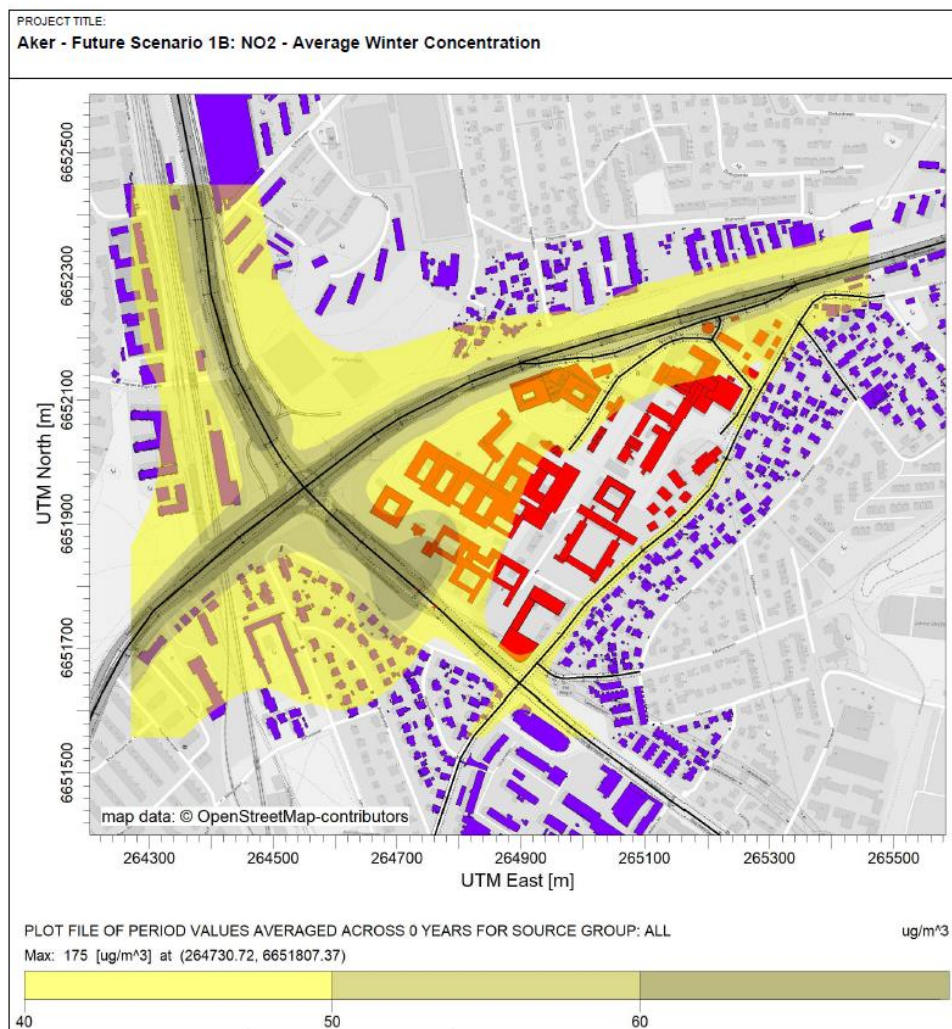
Figur V1- 6. Luftsonkart som viser modellerte konsentrasjoner av nitrogendioksid (NO 2 ) for området ved Aker sykehus ved 2-3 meters høyde for planalternativ 1B med støyskjerm mot Ring 3. Gul sone tilsvarer overskridelse av grensen på 40 µg/m 3 vintermiddel, i henhold til Retningslinje for behandling av luftkvalitet i arealplanlegging (T-1520) (Miljøverndepartementet, 2012).
