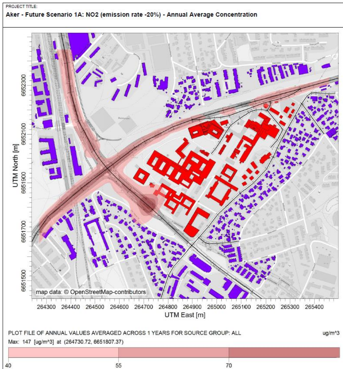
Figur 39. Luftsonekart som viser modellerte konsentrasjoner av nitrogendioksid (NO 2 ) for området ved Aker sykehus ved 2-3 meters høyde for planalternativ 1A med 20% redusert utslipp. Rød sone tilsvarer overskridelse av grensen på 40 µg/m 3 årsmiddel, i henhold til Retningslinje for behandling av luftkvalitet i arealplanlegging (T-1520) (Miljøverndepartementet, 2012).
