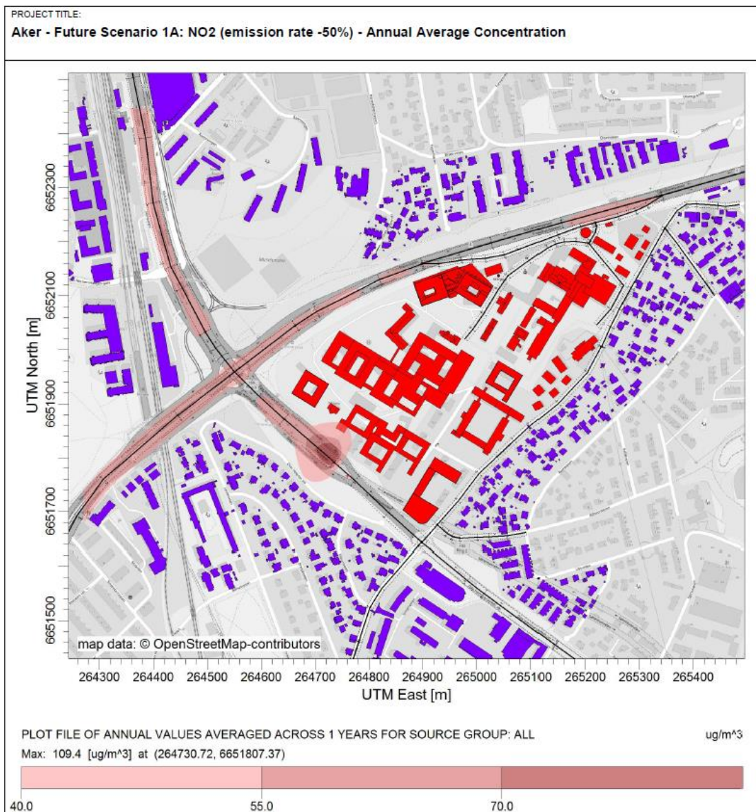
Figur 40. Luftsoneskart som viser modellerte konsentrasjoner av nitrogendioksid (NO 2 ) for området ved Aker sykehus ved 2-3 meters høyde for planalternativ 1A med 50% redusert utslipp. Rød sone tilsvarer overskridelse av grensen på 40 µg/m 3 årsmiddel, i henhold til Retningslinje for behandling av luftkvalitet i arealplanlegging (T-1520) (Miljøverndepartementet, 2012).
