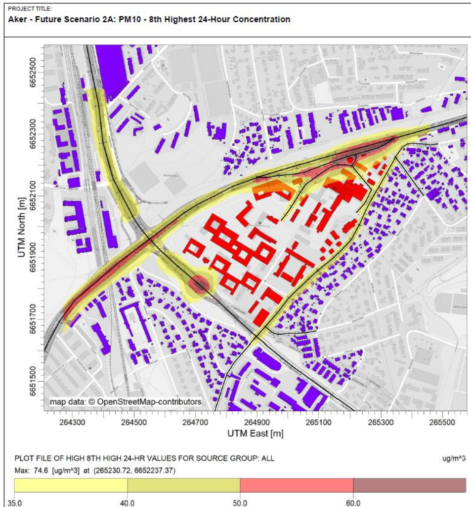
Figur V1- 7. Luftsonkart som viser modellerte konsentrasjoner av svevestøv (PM 10 ) for området ved Aker sykehus ved 2-3 meters høyde for planalternativ 2A med støyskjerm mot Ring 3. Gul og rød sone for PM 10 tilsvarer maksimum 7 overskridelser av grensene på henholdsvis 35 og 50 µg/m 3 , i henhold til Retningslinje for behandling av luftkvalitet i arealplanlegging (T-1520) (Miljøverndepartementet, 2012)
