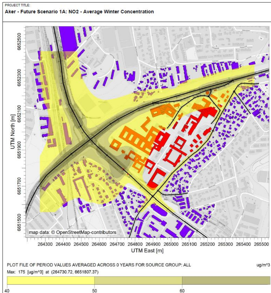
Figur V1- 3. Luftsonkart som viser modellerte konsentrasjoner av nitrogendioksid (NO 2 ) for området ved Aker sykehus ved 2-3 meters høyde for planalternativ 1A med støyskjerm mot Ring 3. Gul sone tilsvarer overskridelse av grensen på 40 µg/m 3 vintermiddel, i henhold til Retningslinje for behandling av luftkvalitet i arealplanlegging (T-1520) (Miljøverndepartementet, 2012).
