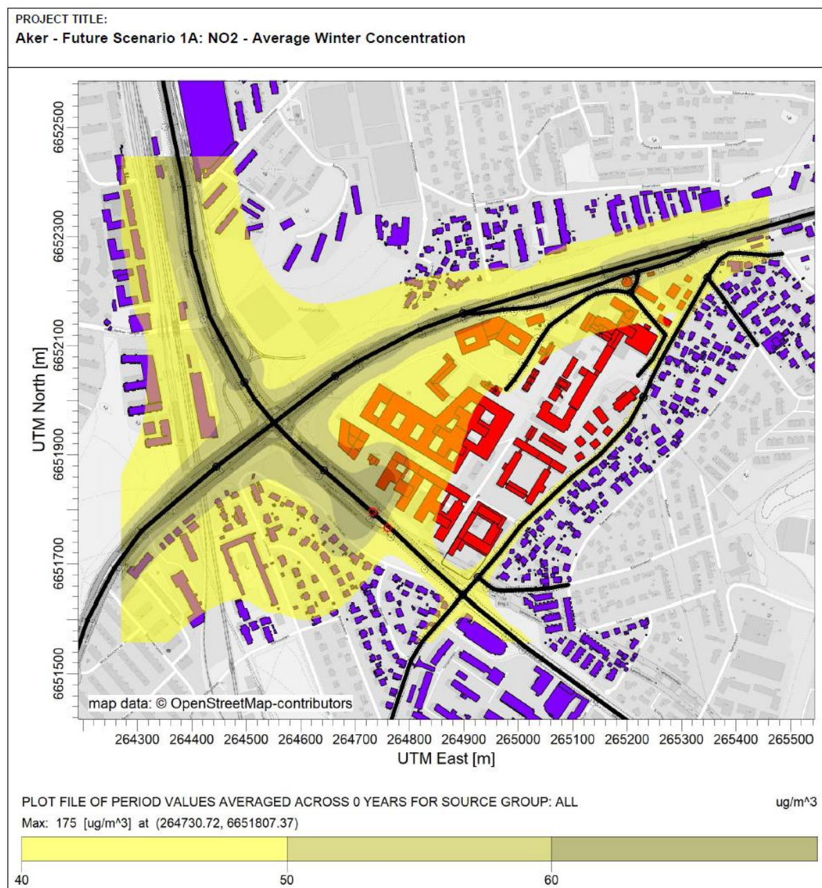
Figur 29. Luftsonkart som viser modellerte konsentrasjoner av nitrogendioksid (NO 2 ) for området ved Aker sykehus ved 2-3 meters høyde for planalternativ 1A. Gul sone tilsvarer overskridelse av grensen på 40 µg/m 3 vintermiddel, i henhold til Retningslinje for behandling av luftkvalitet i arealplanlegging (T-1520) (Miljøverndepartementet, 2012).
