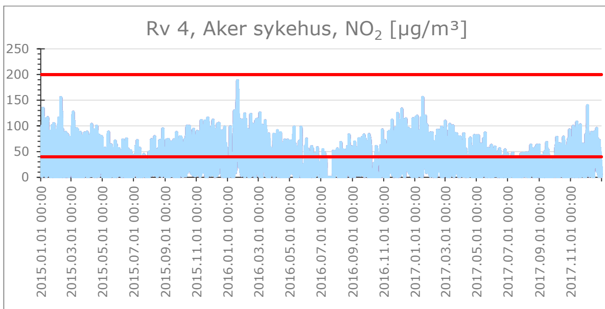
Figur 14. NO 2 -konsentrasjoner på timebasis fra RV4 Aker sykehus målestasjon. (Norsk institutt for luftforskning (NILU); Statens vegvesen; Miljødirektoratet, 2019)
