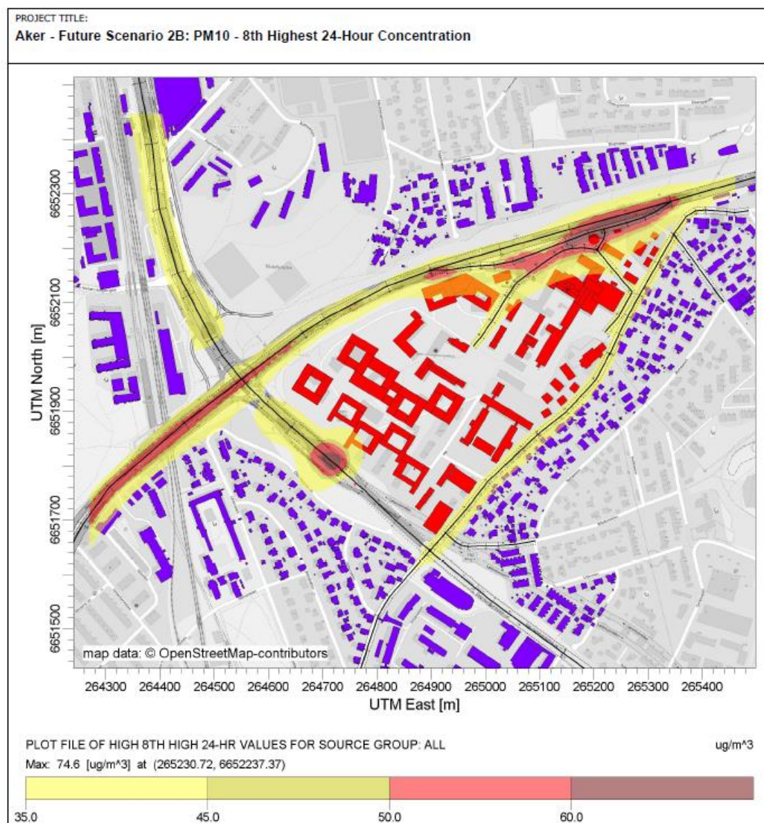
Figur 36. Luftsonekart som viser modellerte konsentrasjoner av svevestøv ( \text{PM}_{10} ) for området ved Aker sykehus ved 2-3 meters høyde for planalternativ 2B. Gul og rød sone for \text{PM}_{10} tilsvarer maksimum 7 overskridelser av grensene på henholdsvis 35 og 50 \mu\text{g}/\text{m}^3 , i henhold til Retningslinje for behandling av luftkvalitet i arealplanlegging (T-1520) (Miljøverndepartementet, 2012).
