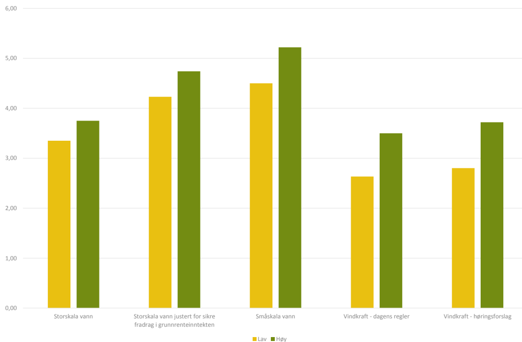
Figur 2: Bedriftsøkonomiske investeringsgrenser for vindkraft- og vannkraftprosjekter. Kr/kWh
