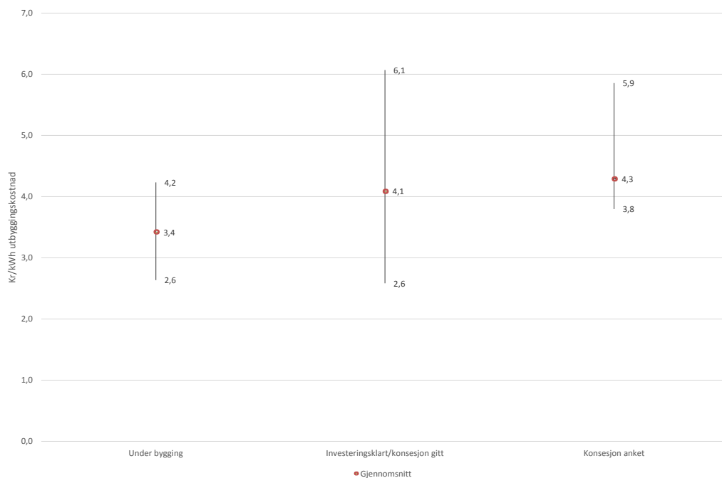
Figur 4: Kostnadsfordeling for småkraftprosjekter pr. kategori. Kr/kWh utbyggingskostnad
