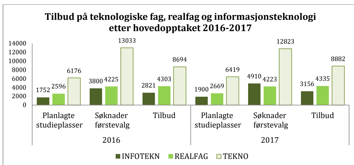
Diagram 8: Tilbudene på teknologiske fag, realfag og informasjonsteknologiske fag 2016-2017
