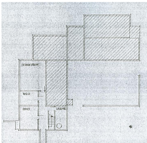
Plantegning kjeller. Opphavsrett: Statsbygg.
