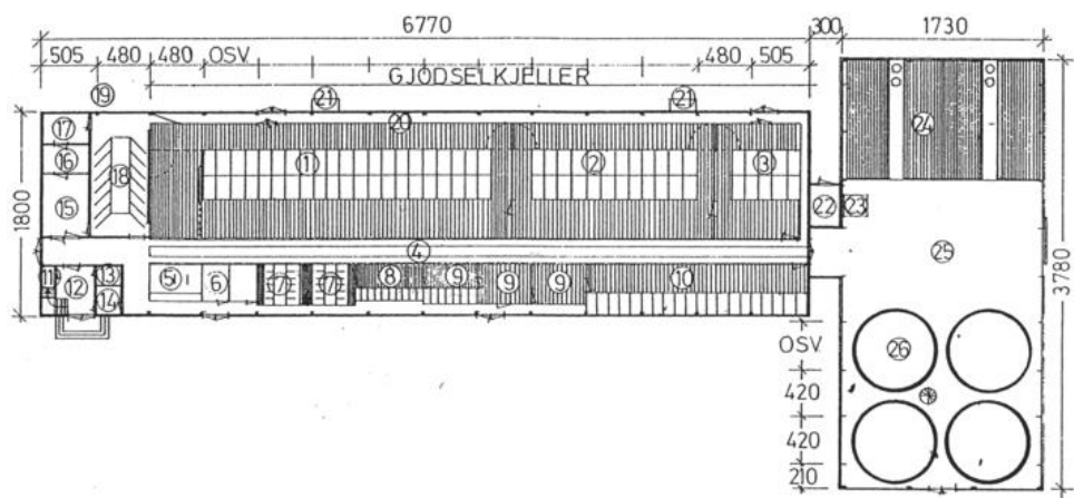
Grunnplan. Foto: Akershus Landbrukssekskap. Opphavsrett: Statsbygg.
