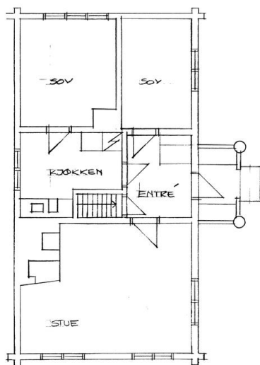
Plan 1. etasje. Foto: Opptegnet av 4B Arkitekter. Opphavsrett: Statsbygg.
