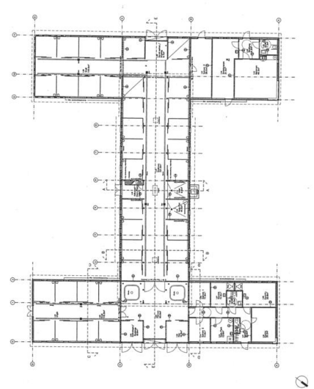
Plantegning stallbyggingen. Foto: Kvernaas Arkitekter. Opphavsrett: Statsbygg.
