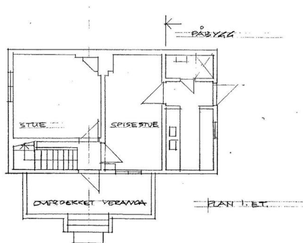
Plan 1. etasje. Foto: 4B Arkitekter. Opphavsrett: Statsbygg.
