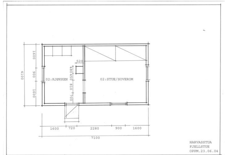
Plantegning. Opphavsrett: Statsbygg.
