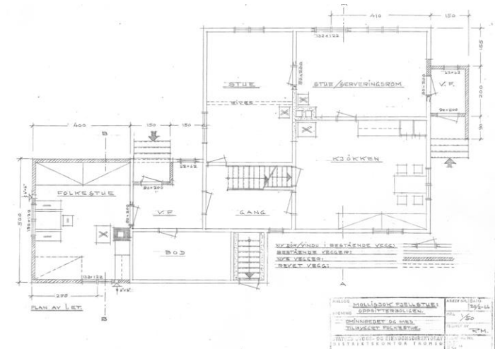
Plantegning for 1. etasje fra 1966. Opphavsrett: Statsbygg.
