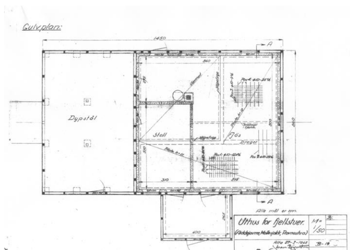
Plan 1 etg. Signert Johan Bjørnstad. Opphavsrett: Statsbygg.
