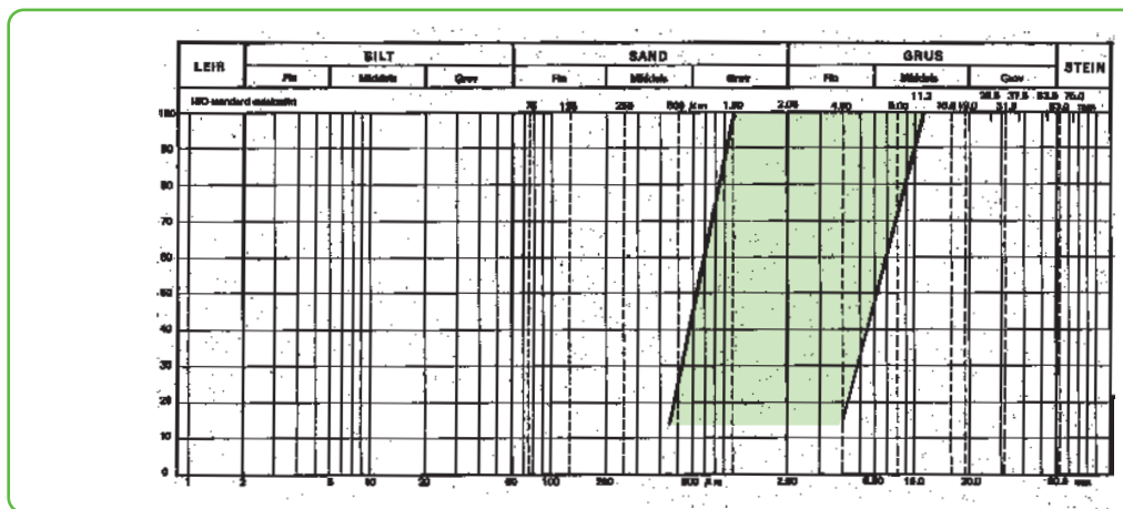
Figur 1 Eksempel på grensekurver for drens masse.
