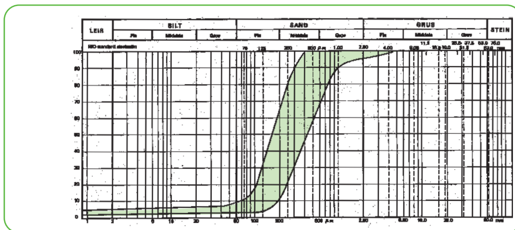
Figur 3 Anbefalt vekstmasse ligger i det skraverte område.
