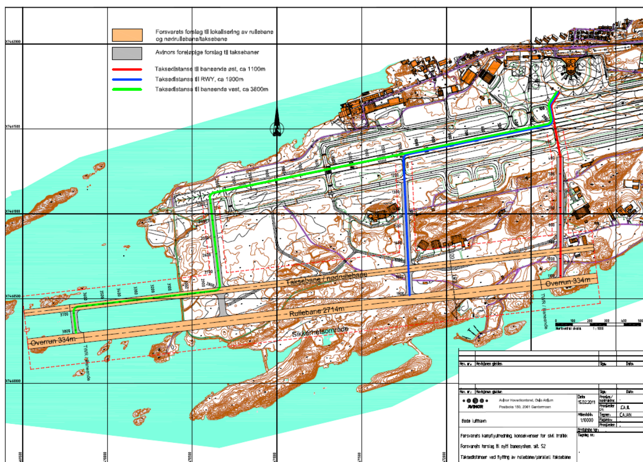
Figur 31 – Antatte takseveier i Bodø ved kampflybase
