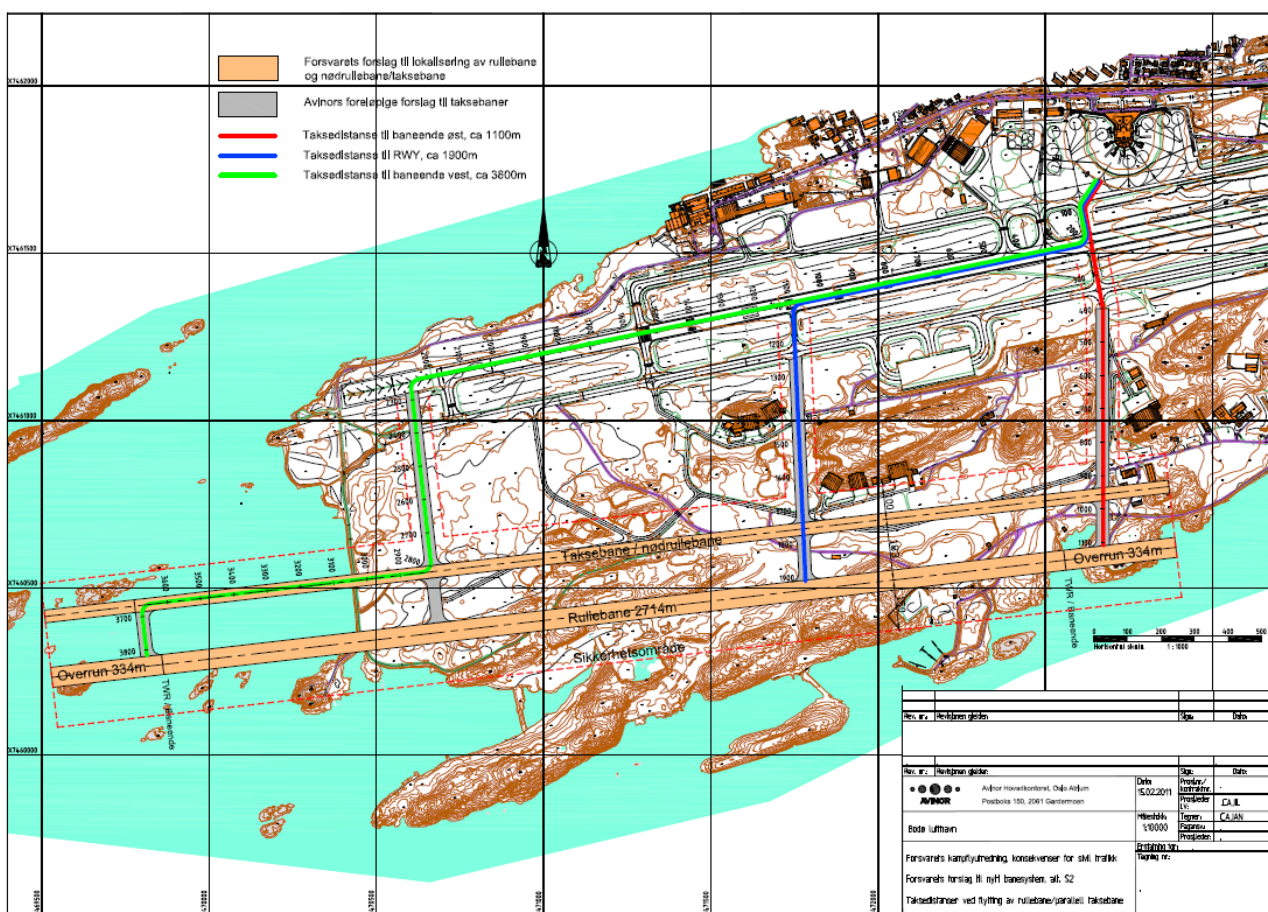
Figur 5 – Skisse som illustrerer takseavstander fra terminalområdet til ny runnebane
