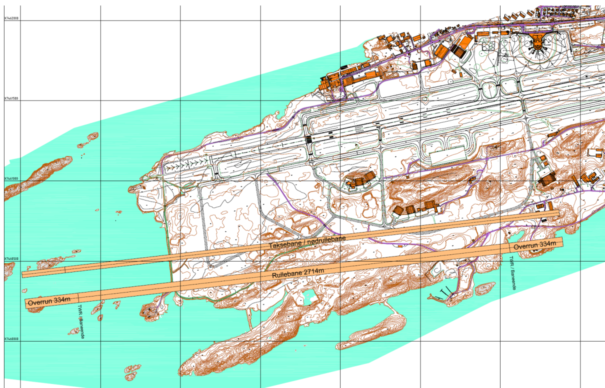
Figur 1 - Nytt banesystem om kampflybase i Bodø 5
