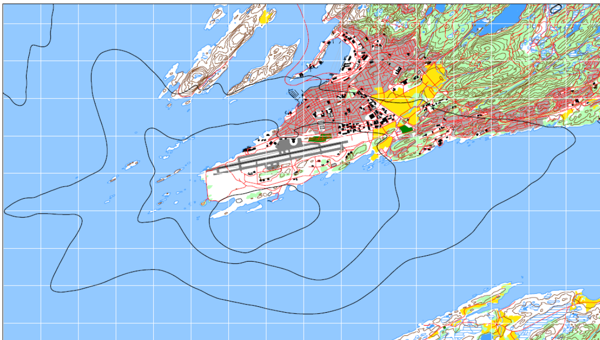
Figur 29 – L_{den} for total trafikk i 2016. 27
