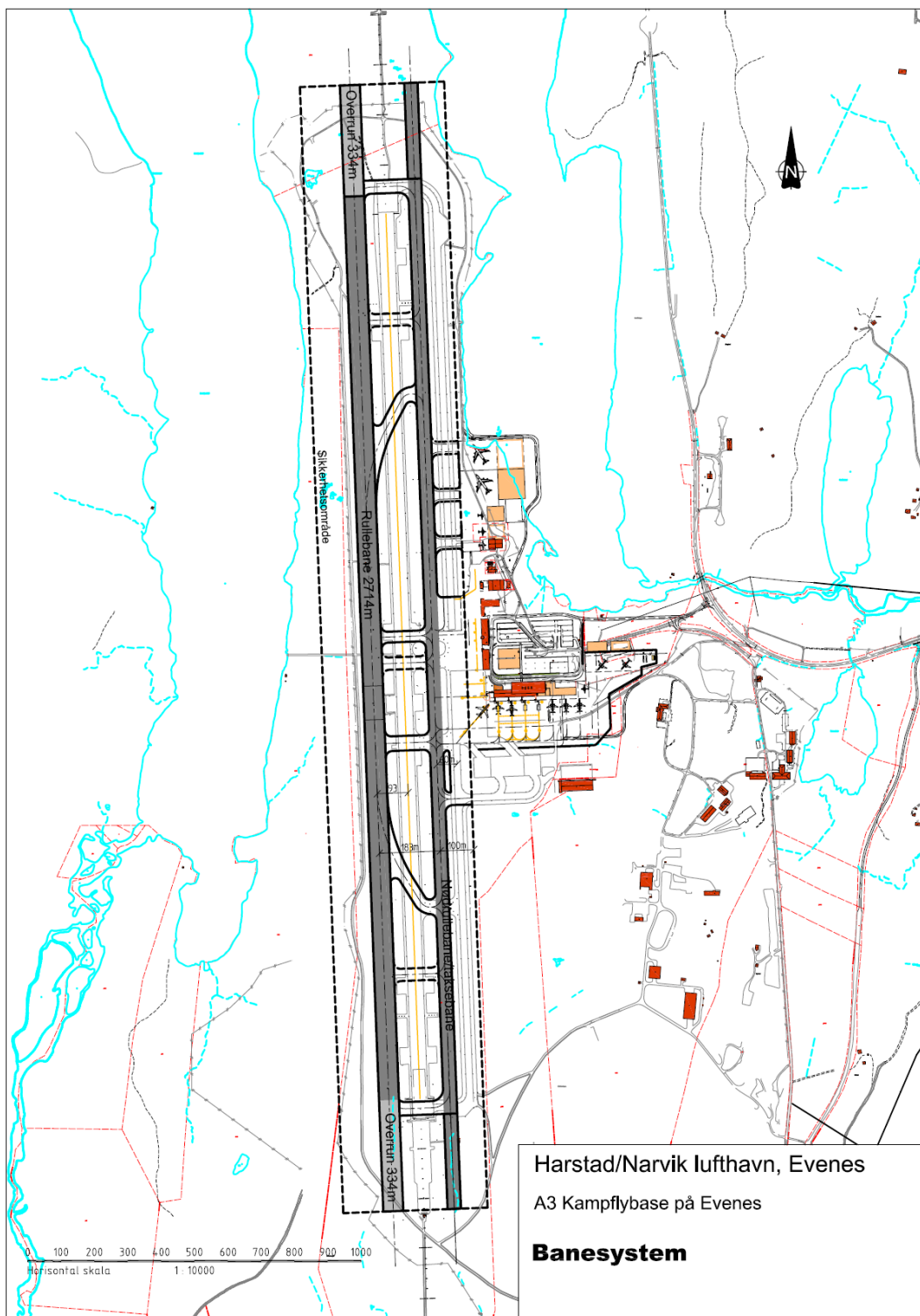
Figur 8 - Nytt banesystem på Evenes som kampflybase
