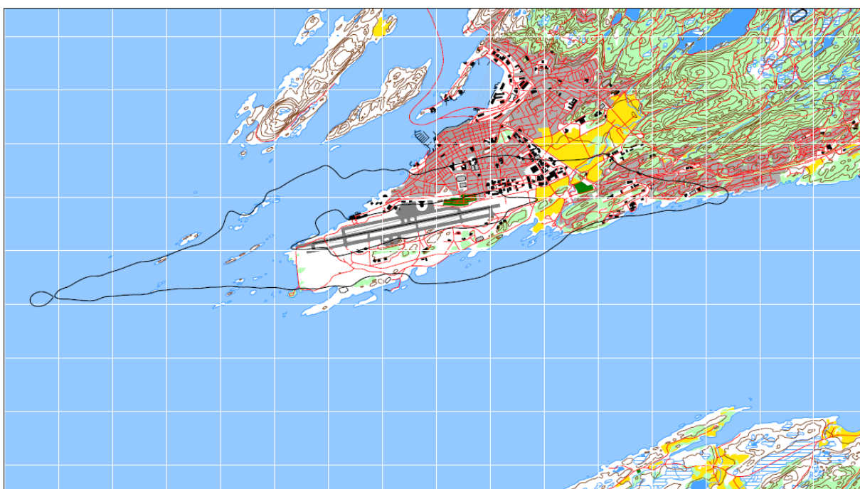
Figur 30 - L_{den} for sivil trafikk i 2016.
