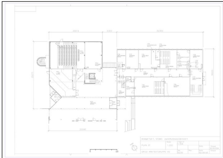
Opprinnelig plan 1. etg. 1994-bygget t v i planen. Opphavsrett: Statsbygg
