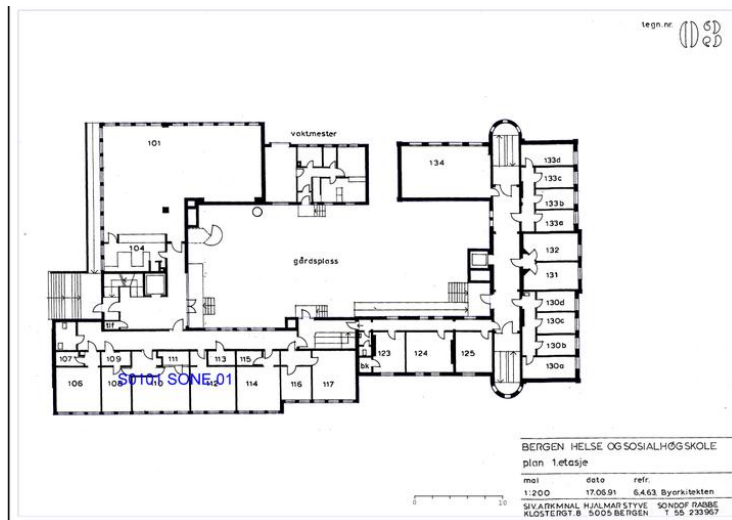
Plan 1.etg Opphavsrett: Statsbygg v/Styve og Rabbe
