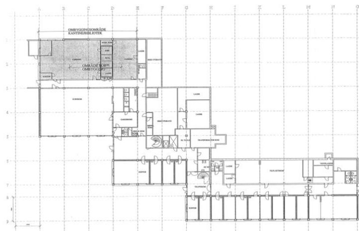
Plan første etasje med ombygging Foto: Scannet fra tegningsarkiv Opphavsrett: Mellbye arkitekter as
