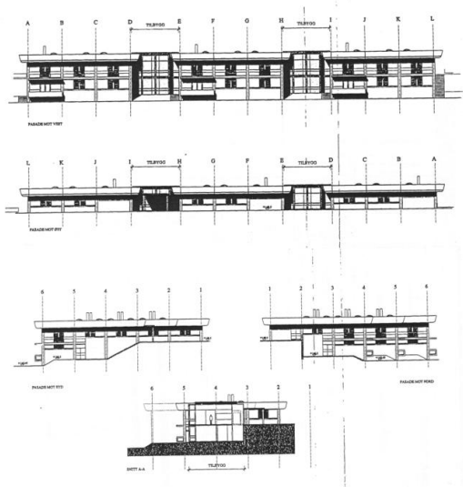
Fasader gul, grønn og rødstua med nye mellombygg Foto: Scannet fra tegningsarkiv Opphavsrett: Mellbye arkitekter as Gultstua, Grønnstua og Rødstua sett fra vest Opphavsrett: Statsbygg.
