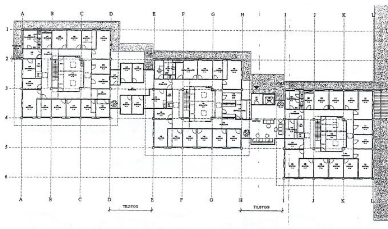
Plan 1. etasje Gul, grønn og rød med nye mellombygg Foto: Scannet fra tegningsarkiv Opphavsrett: Mellbye arkitekter as
