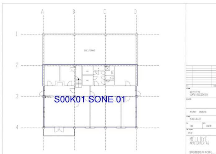
Plan kjeller etasje. Vannmerke fra Statsbyggs eiendomsdatabase Propman er på tegningen. Foto: Scannet fra Statsbyggs tegningsarkiv Opphavsrett: Mellbye arkitekter AS
