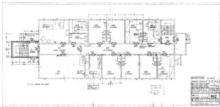
Plantegning opprinnelig utforming av 1. etasje. Opphavsrett: Statsbygg.
