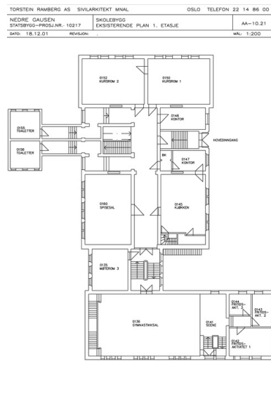
Plantegning 1.etg. Opphavsrett: Statsbygg.
