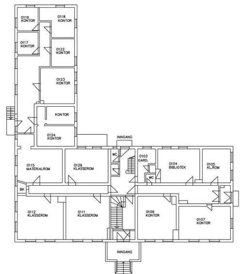
Plantegning 1.etg. Opphavsrett: Statsbygg.
