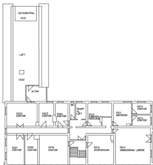
Plantegning 2.etg. Opphavsrett: Statsbygg.
