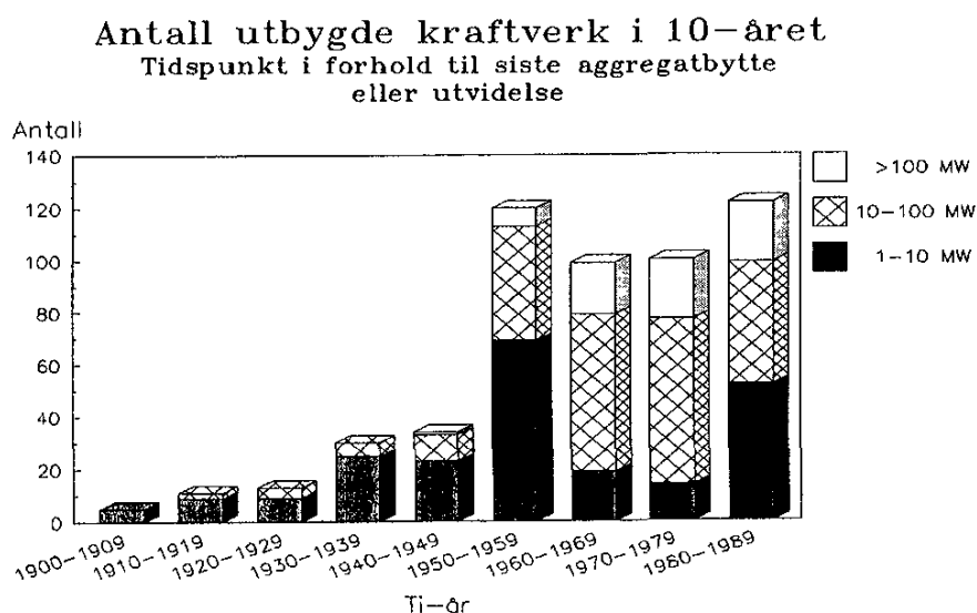
Figur 1. Eksisterende kraftstasjoner fordelt etter alder og størrelse (NVE, ER-notat nr. 25/91)
