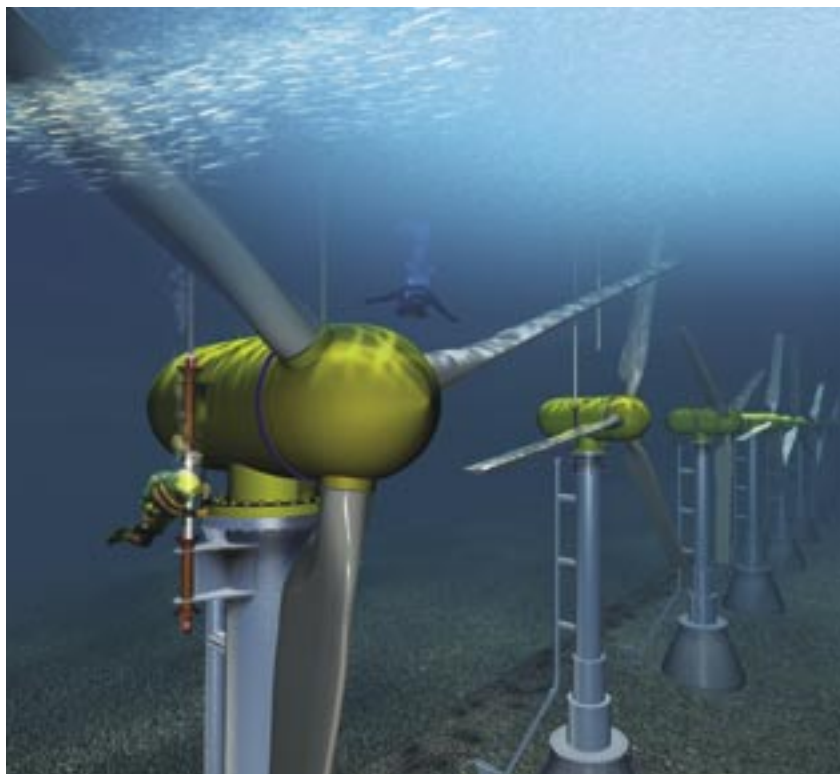
Tidevannskraftverket i Kvaløysundet skal starte kommersiell drift i 2004
