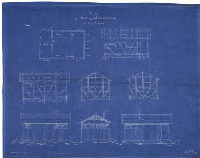
Byggtegning fra Riksarkivet
