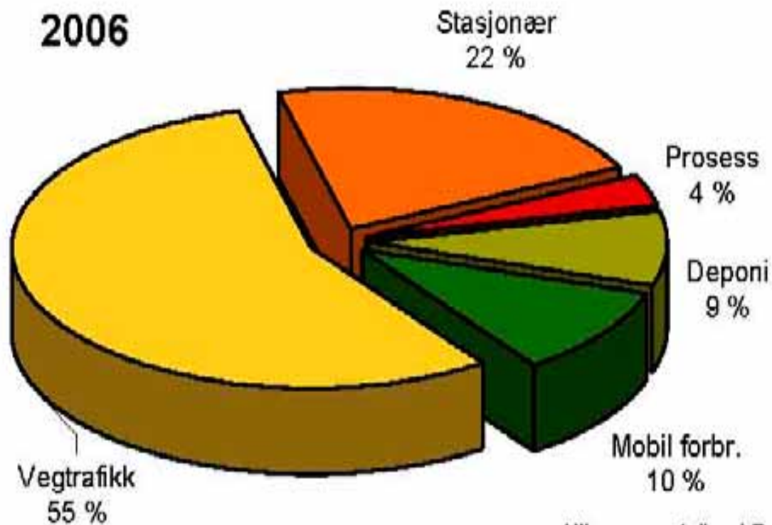
Klimagassutslipp i Bergen 2006 fordelt på kilde
