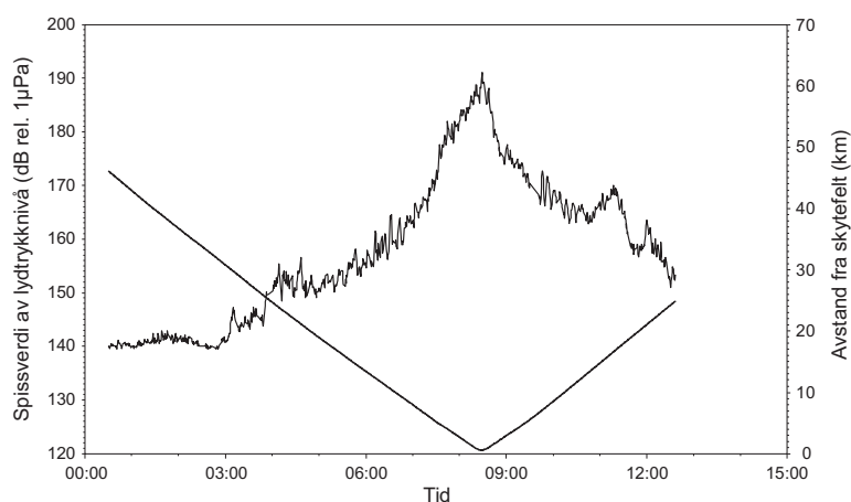
Figur 3.4.1. Lydtrykknivå (spissverdi) fra en seismisk kurslinje i forhold til avstanden fra luftkanonfeltet til målepunktet. Skipet passerte like over en hydrofonrigg som var satt ut på 184 m dyp. Når målingene starten var fartøyet ca. 45 km fra riggen. (Sound pressure level (peak value) from one seismic survey line relative to the distance from the air-gun array. The vessel passed close to a hydrophone rig deployed at 184 m depth. When the measurements started the vessel was about 45 km from the rig.)
