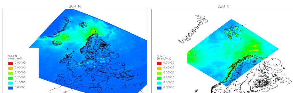
Figur 6.1: Beregnet total årsavsetning av nitrogen fra petroleumsbildene til hele EMEP-området (venstre) og det mellomste modellområdet (høyre). Enhet: mg N/m 2 .
