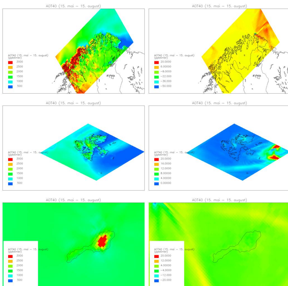
Figur 6.7: Beregnet 3-mnd AOT40-verdi for ozon (relevant for planter) for tre regioner for bakgrunnssituasjonen (venstre) og forskjellen pga petroleumsutslippene (høyre). Legg merke til at skalaen er forskjellig. Enhet: ppb-timer. Grenseverdi: 3000.
