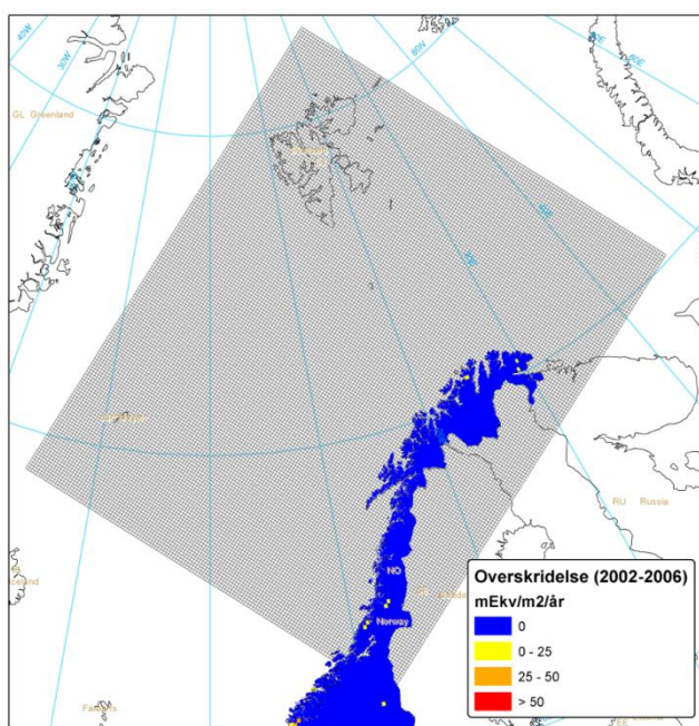
Figur 8.4: Overskridelse av tålegrensen for forsurening av vann, beregnet med SSWC_{oaa} modellen og dagens avrenning av nitrogen, gitt avsetning av nitrogen og svovel som gjennomsnitt for 2002-2006 (Larssen et al. 2008). Influensområdet som er vurdert i denne rapporten er skravert.
