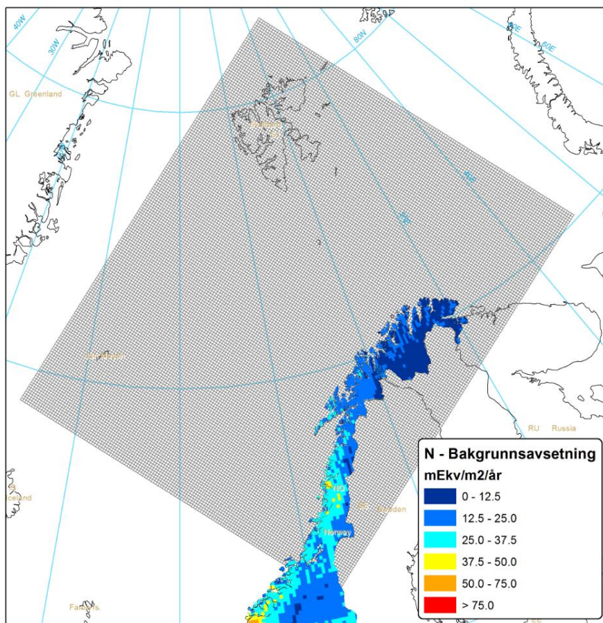
Figur 8.6: Bakgrunnsavsetning av N uten petroleumsaktivitet ved Jan Mayen og i Barentshavet.
