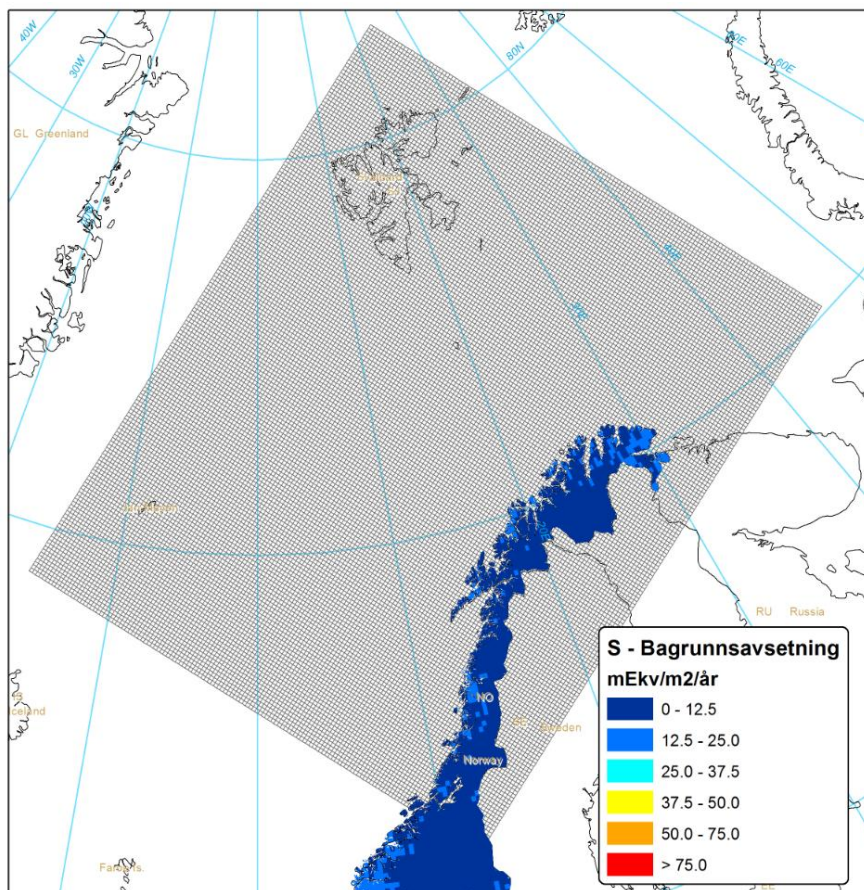
Figur 8.5: Bakgrunnsavsetning av S uten petroleumsaktivitet ved Jan Mayen og i Barentshavet.
