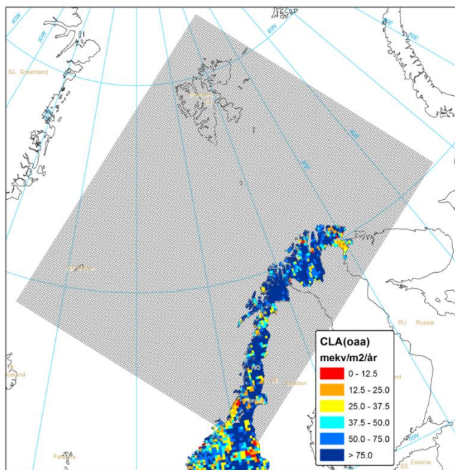
Figur 8.3: Tålegrenser for forsurening av overflatevann hvor det er tatt hensyn til organiske syrer ( CLA_{oaa} ). Influensområdet som er vurdert i denne rapporten er skravert.
