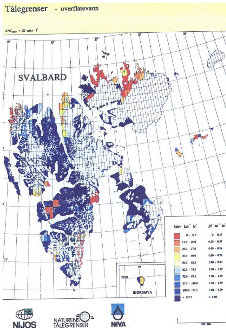
Figur 8.1: Tålegrenser for tilførsler av sterke syrer på Svalbard. Tålegrensene er beregnet på grunnlag av \text{ANC}_{\text{limit}} = 20 \mu\text{ekv/l} . Rød – orange – gul – blå viser økende tålegrenser. Hvite felt er breer og isdekket land. Grå felter er nunatak og mindre øyer som ikke er prøvetatt. (Lien et al 1993).
