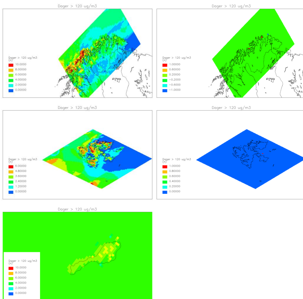
Figur 6.8: Beregnet N120-verdi for ozon (relevant for helse) for tre regioner for bakgrunssituasjonen (venstre) og forskjellen pga petroleumsutslippene (høyre). Skalaen er forskjellig. Det var ingen forskjell for Jan Mayen med petroleumsutslippene, så den figuren er derfor utelatt. Enhet: antall dager. Grenseverdi: 25 ("target value") og 0 ("long-term objective").
