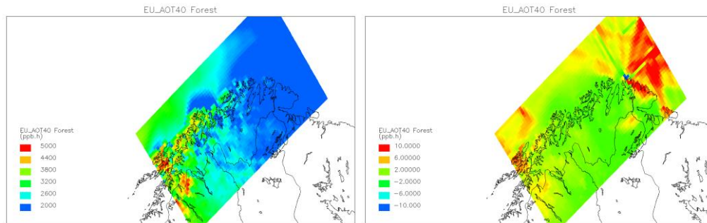
Figur 6.6: Beregnet 6-mnd AOT40-verdi for ozon (relevant for skog) for Nord-Norge for bakgrunnssituasjonen (venstre) og forskjellen pga petroleumsutslippene (høyre). Legg merke til at skalaen er forskjellig. Enhet: ppb-timer. Grenseverdi: 5000.
