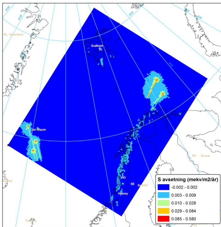
Figur 8.7: Beregnet avsetning av S på grunn av utslipp fra petroleumsvirksomhet ved Jan Mayen og i Barentshavet.
