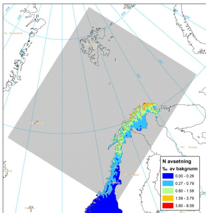
Figur 8.10: Beregnet N-avsetning som ‰ (promille) av bakgrunnsavsetning på grunn av utslipp fra petroleumsvirksomhet ved Jan Mayen og i Barentshavet.
