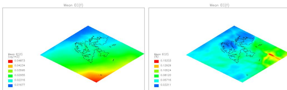
Figur 6.10: Beregnet årsmiddelskonsentrasjon i finfraksjonen av BC på Spitsbergen for bakgrunssituasjonen (venstre) og den relative økningen pga petroleumsutslippene (høyre). Enheter: \mu\text{g}/\text{m}^3 og %.
