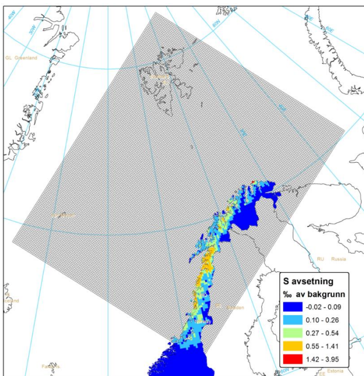
Figur 8.8: Beregnet S-avsetning som ‰ (promille) av bakgrunnsavsetning på grunn av utslipp fra petroleumsvirksomhet ved Jan Mayen og i Barentshavet.
