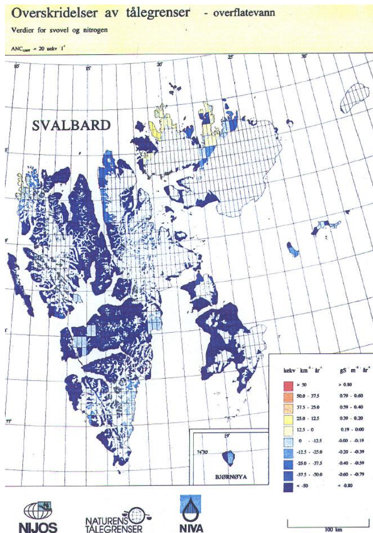
Figur 8.2: Områder på Svalbard der tålegrensene for svovel og nitrogen er overskredet (gul) og ikke er overskredet (blå). Hvite og blå felt som Figur 8.1. (Lien et al 1993).
