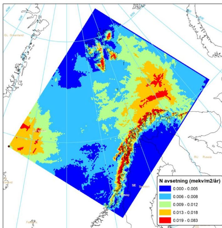
Figur 8.9: Beregnet avsetning av N på grunn av utslipp fra petroleumsvirksomhet ved Jan Mayen og i Barentshavet.
