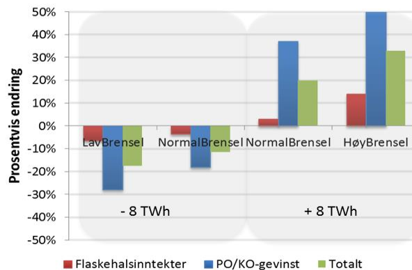
Figur 63: Prosentvise endringer i totale flaskehalsinntekter, PO/KO-gevinst og total nytte sammenlignet med basis 2020 når vi endrer både norsk kraftbalanse med 8 TWh og brenselprisene. For å vise utfallsrommet har vi økt brenselprisene med 20 prosent ved mer positiv kraftbalanse og redusert brenselprisene med 20 prosent ved lavere kraftbalanse. For å kunne vise effektene av høyere brenselpriser har vi også med resultatene der vi bare endrer kraftbalansen med 8 TWh.
